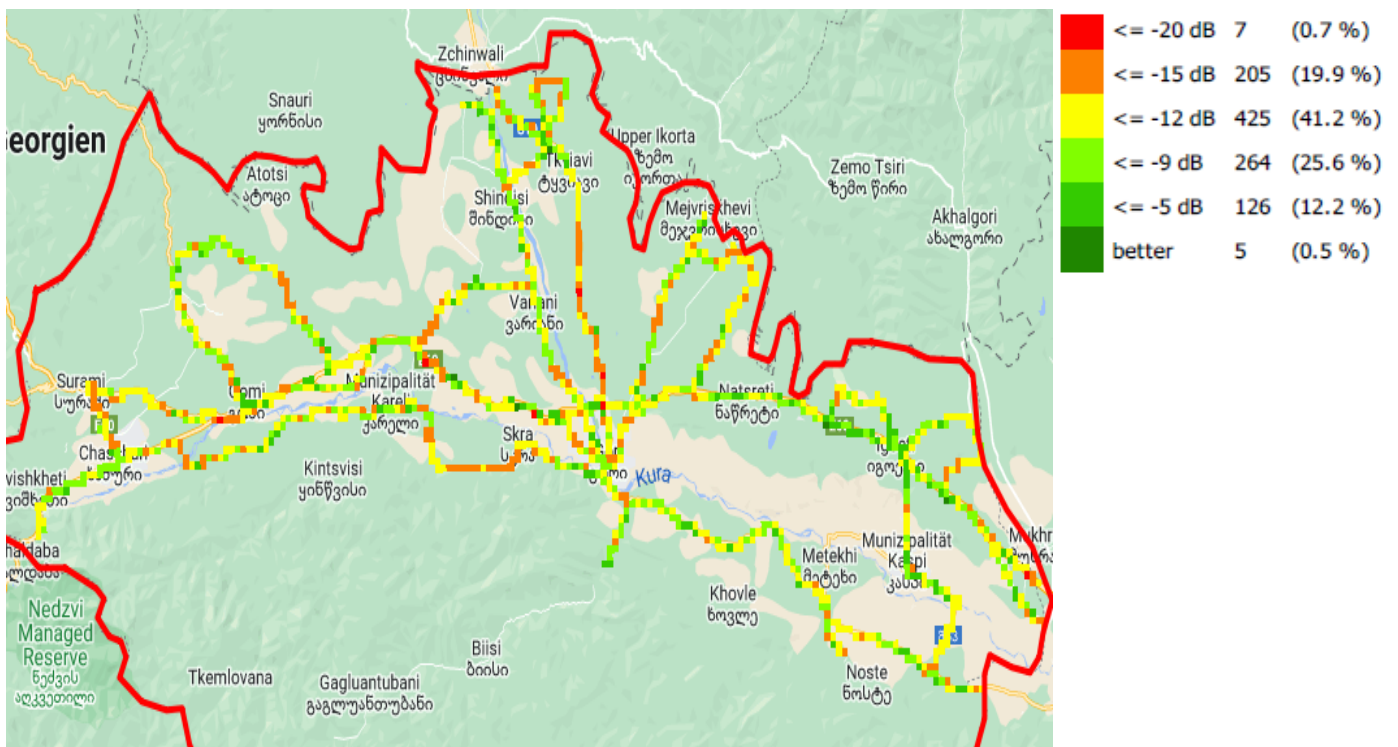
RSRQ, მაგთიკომი
