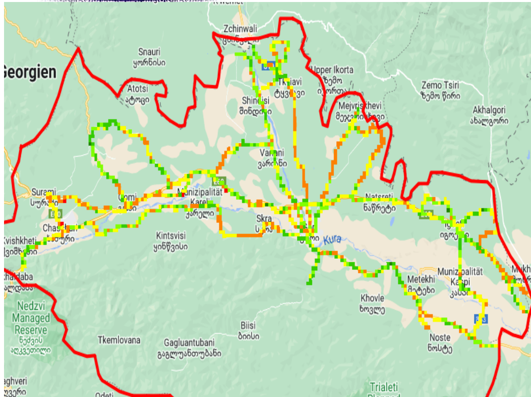
RSRQ, სილქნეტი
