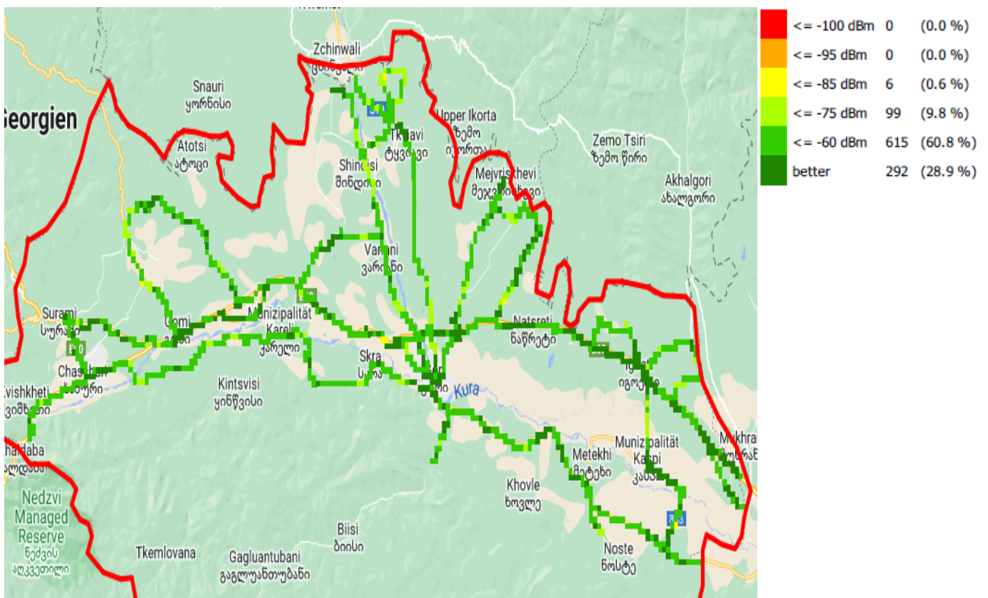
RSCP, მაგთიკომი
