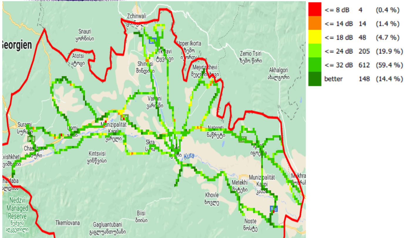
C/I, მაგთიკომი
