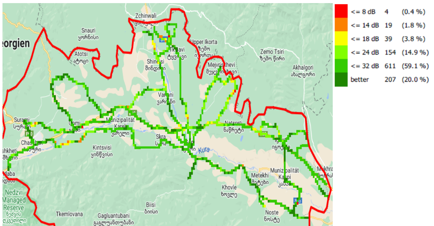
C/I, სილქნეტი
