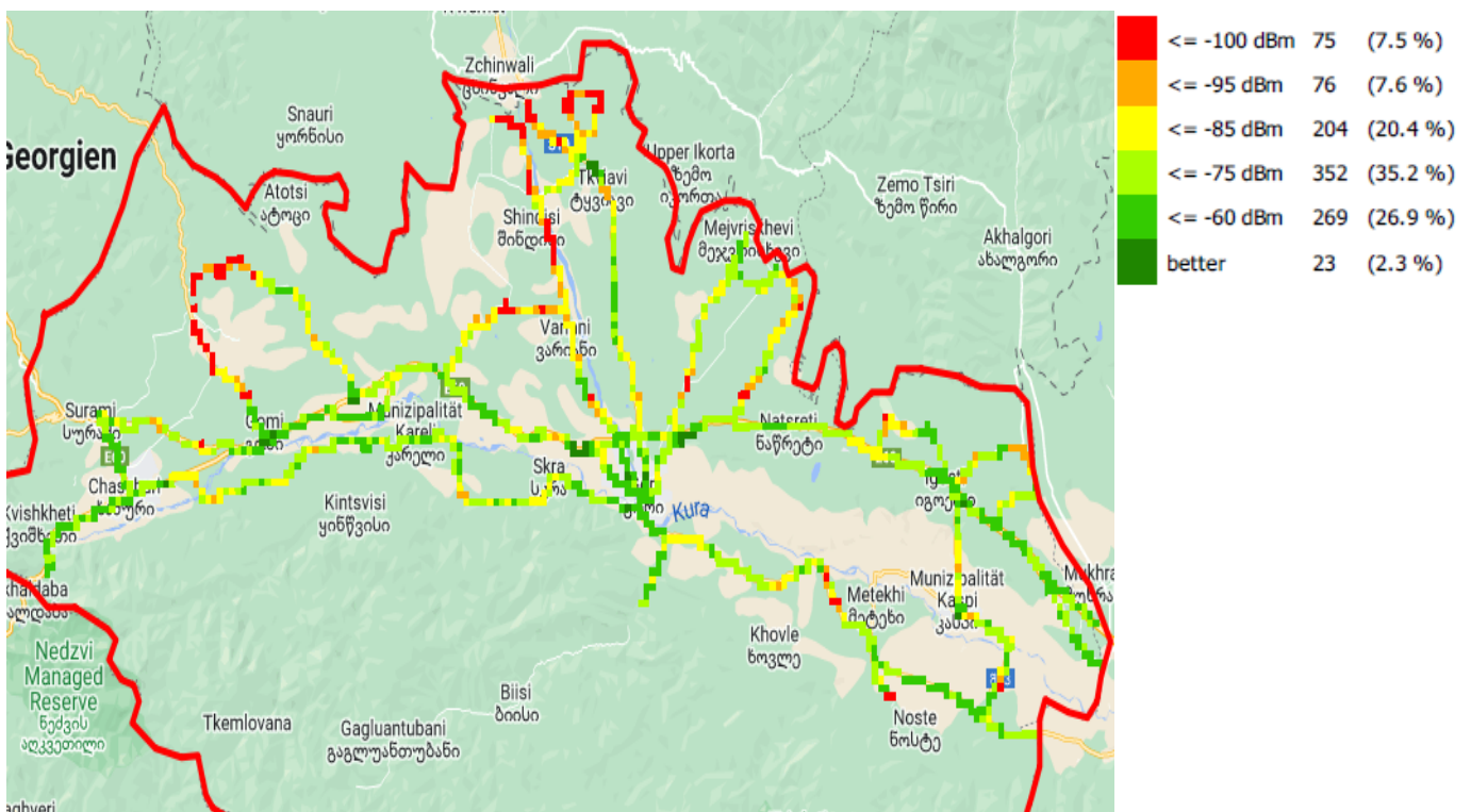
RSCP, ვიონი საქართველო
