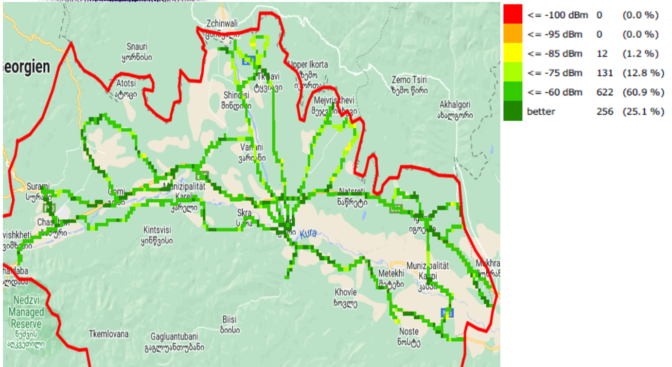
RSCP, სილქნეტი
