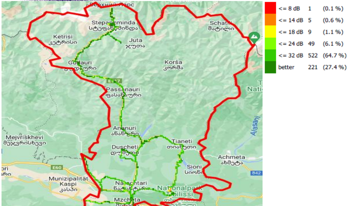
C/I, მაგთიკომი
