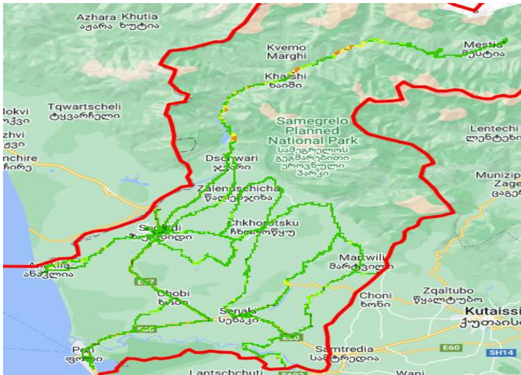
RSRP, მაგთიკომი
