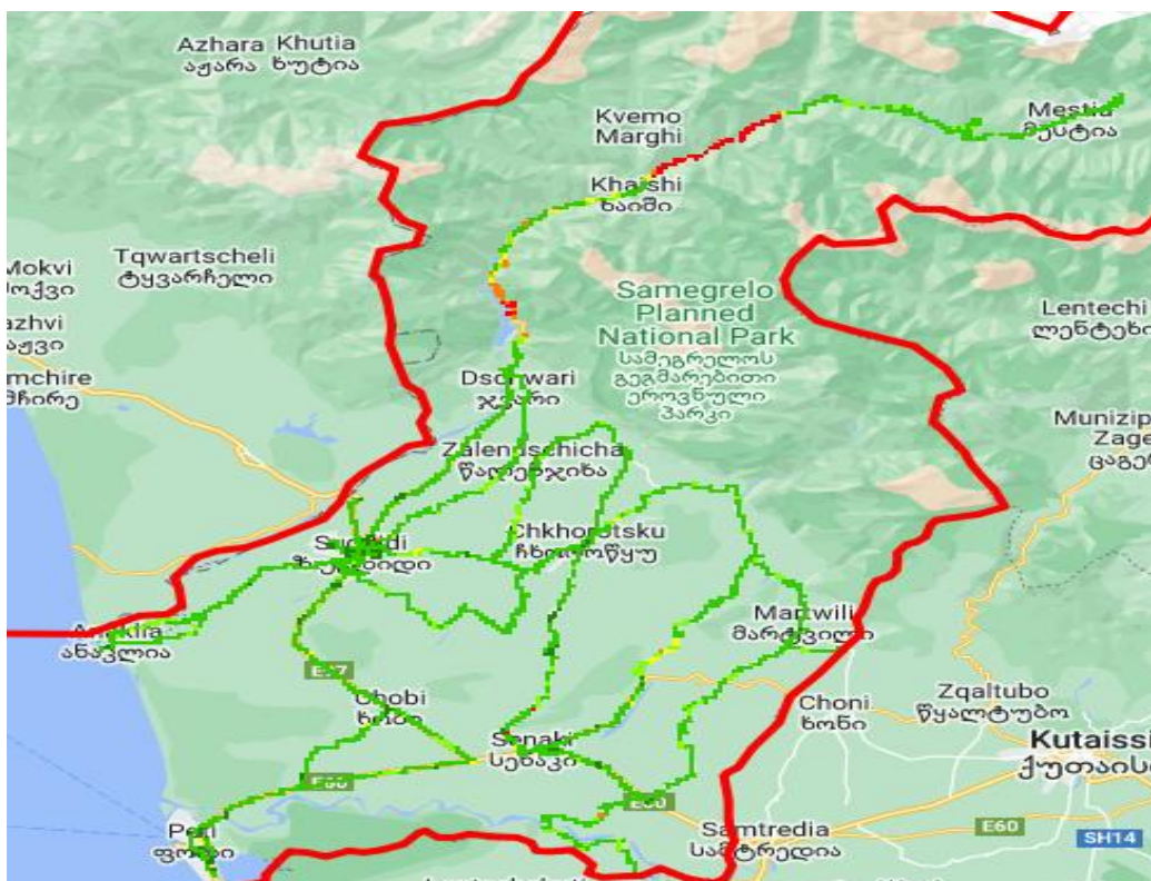
RSRP, სილქნეტი
