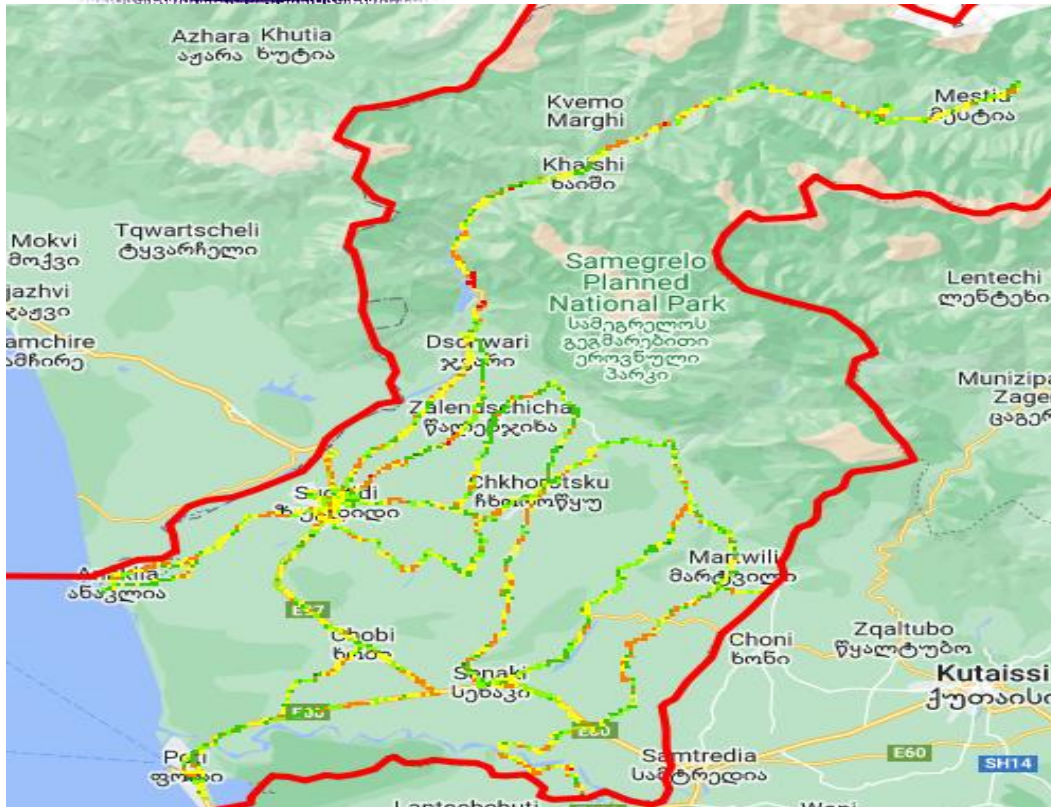
RSRQ სილქნეტი
