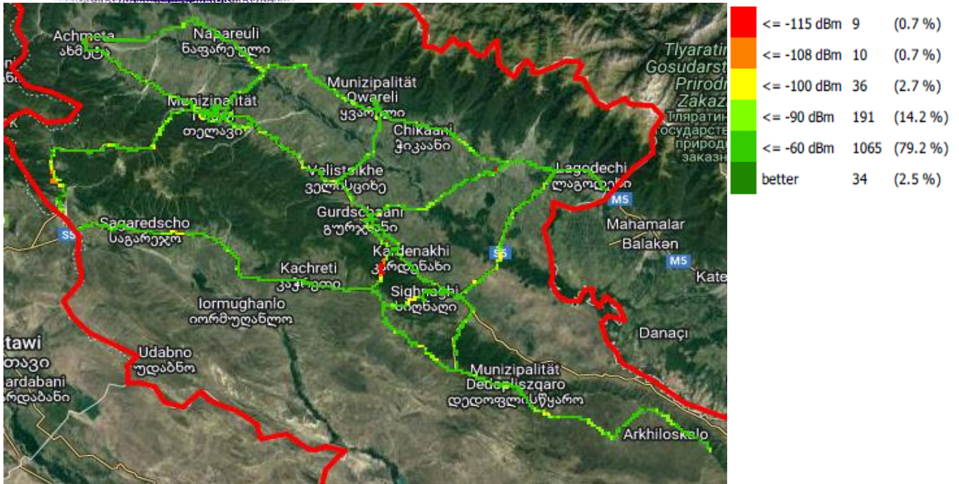
RSRP, ვიონი საქართველო
