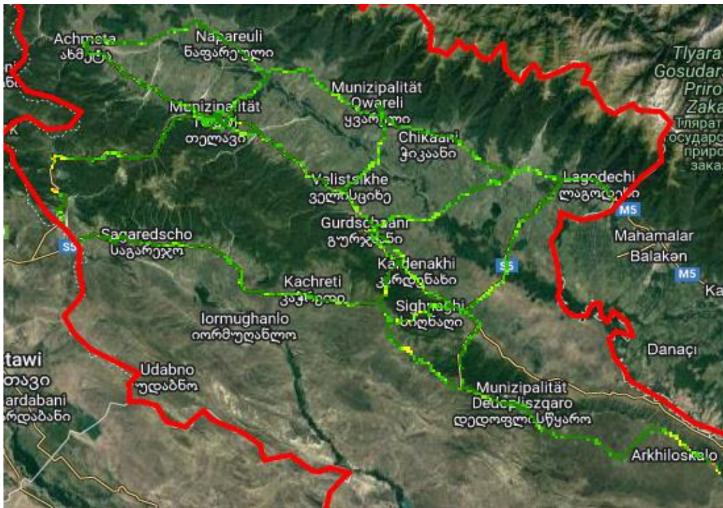
Ec/Io, ვიონი საქართველო
