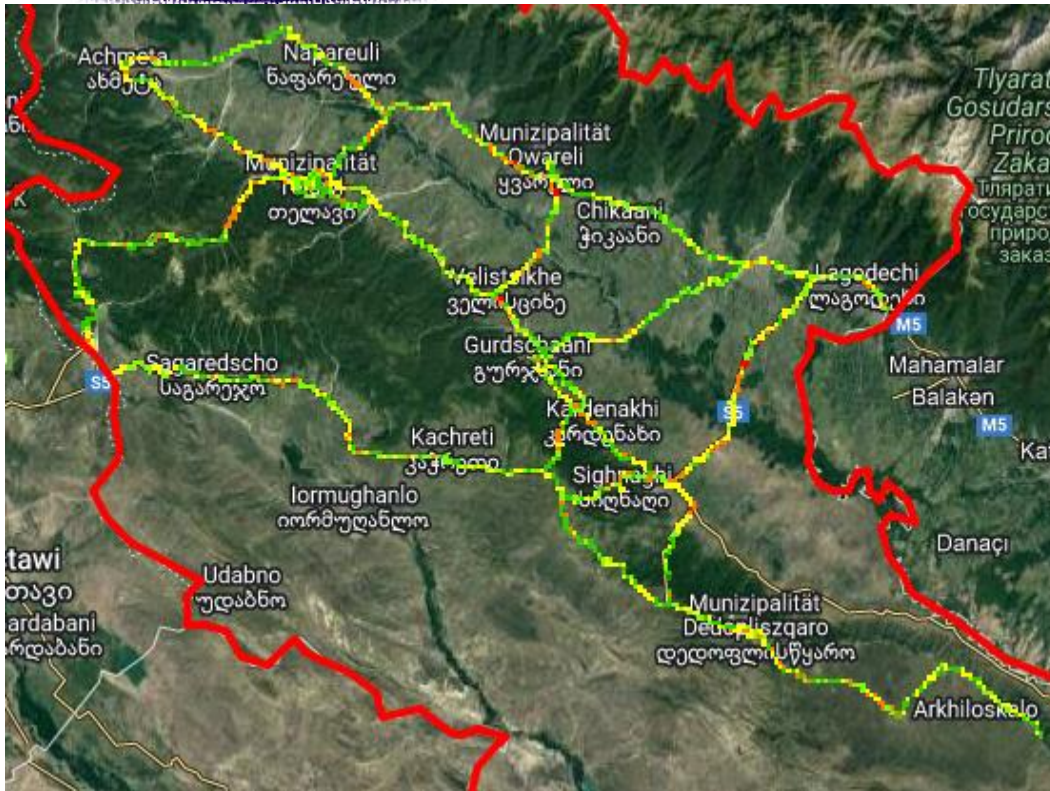
RSRQ სილქნეტი
