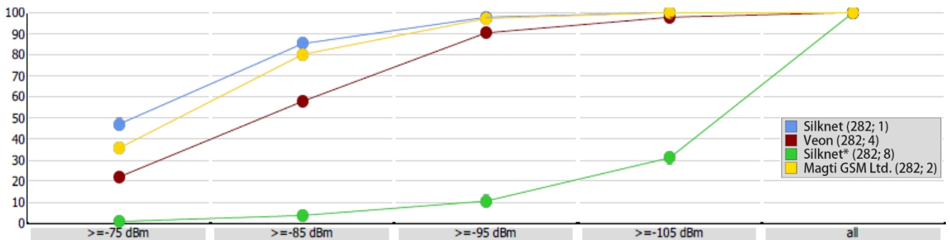
RSRP, ვიონი საქართველო
