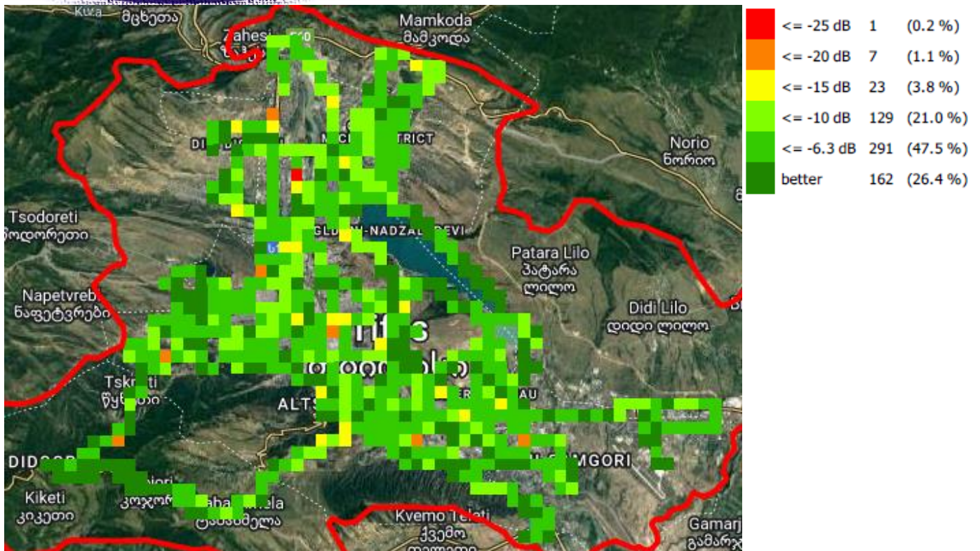
Ec/Io, სოლქნეტი
