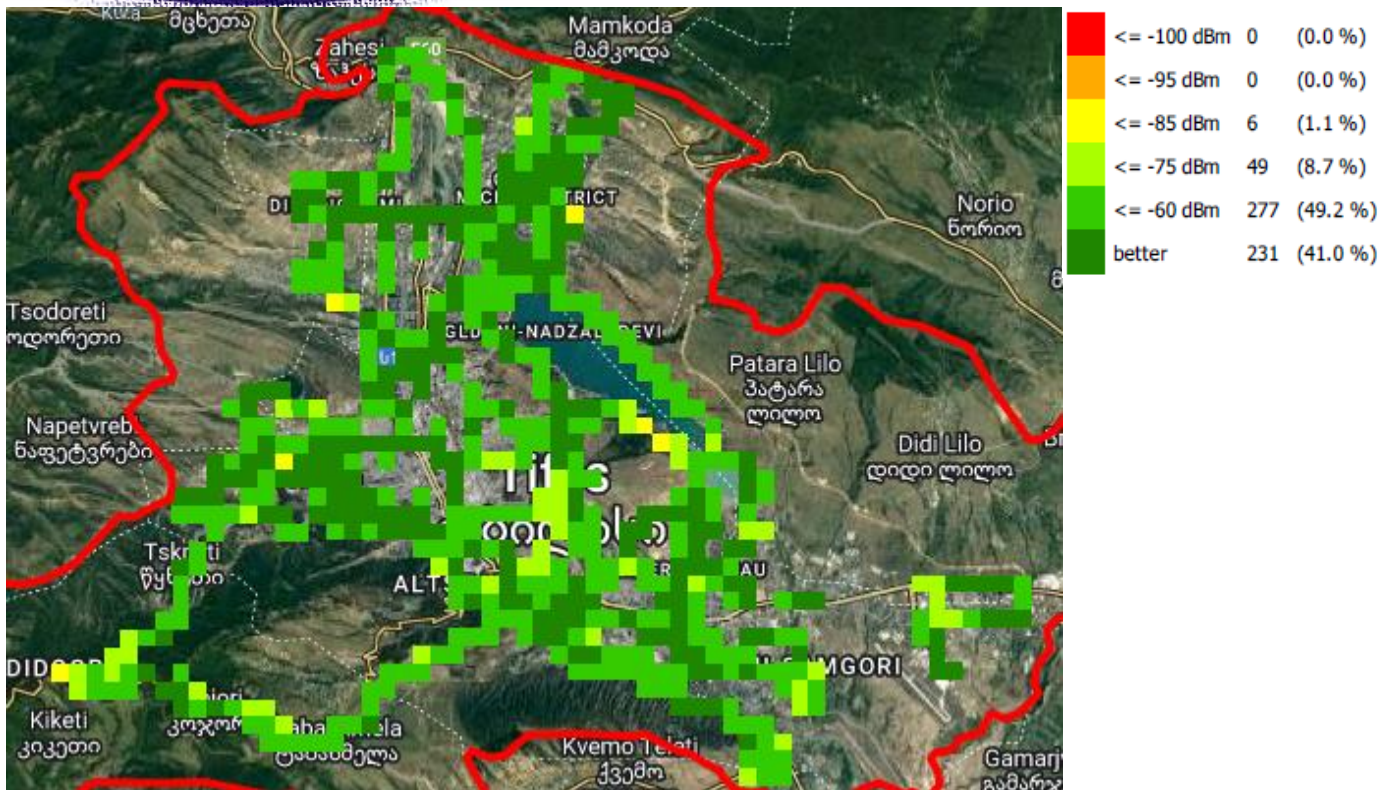
RSCP, მაგთიკომი
