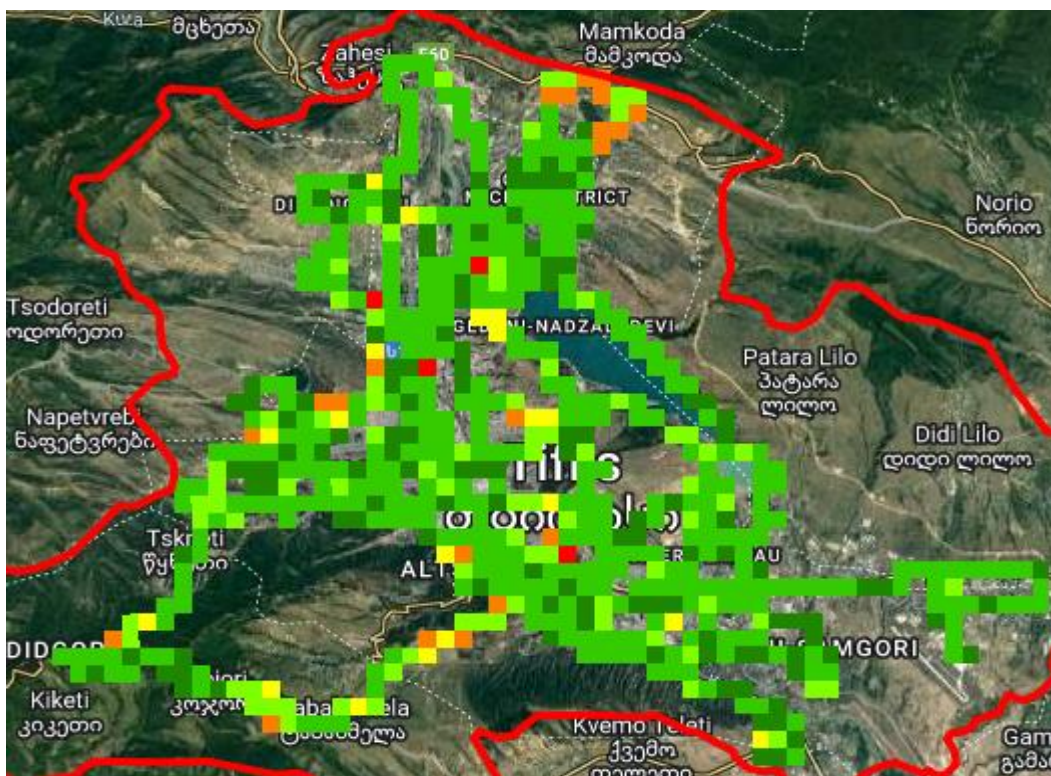
C/I, სილქნეტი
