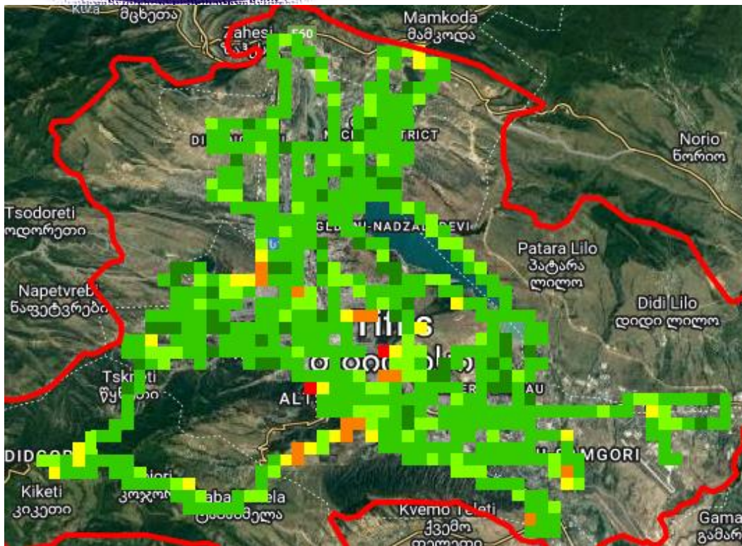
C/I, მაგთიკომი
