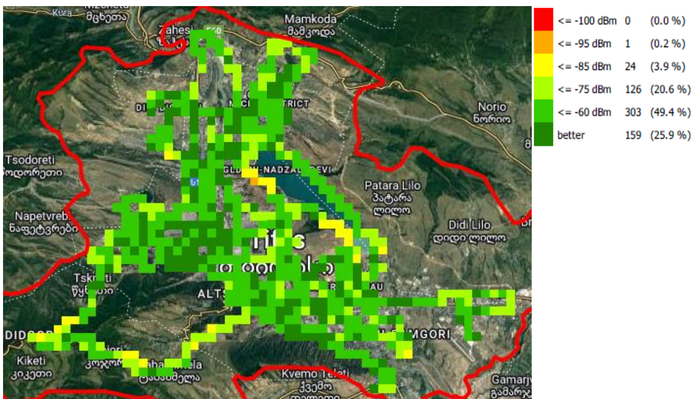
RSCP, სილენტი
