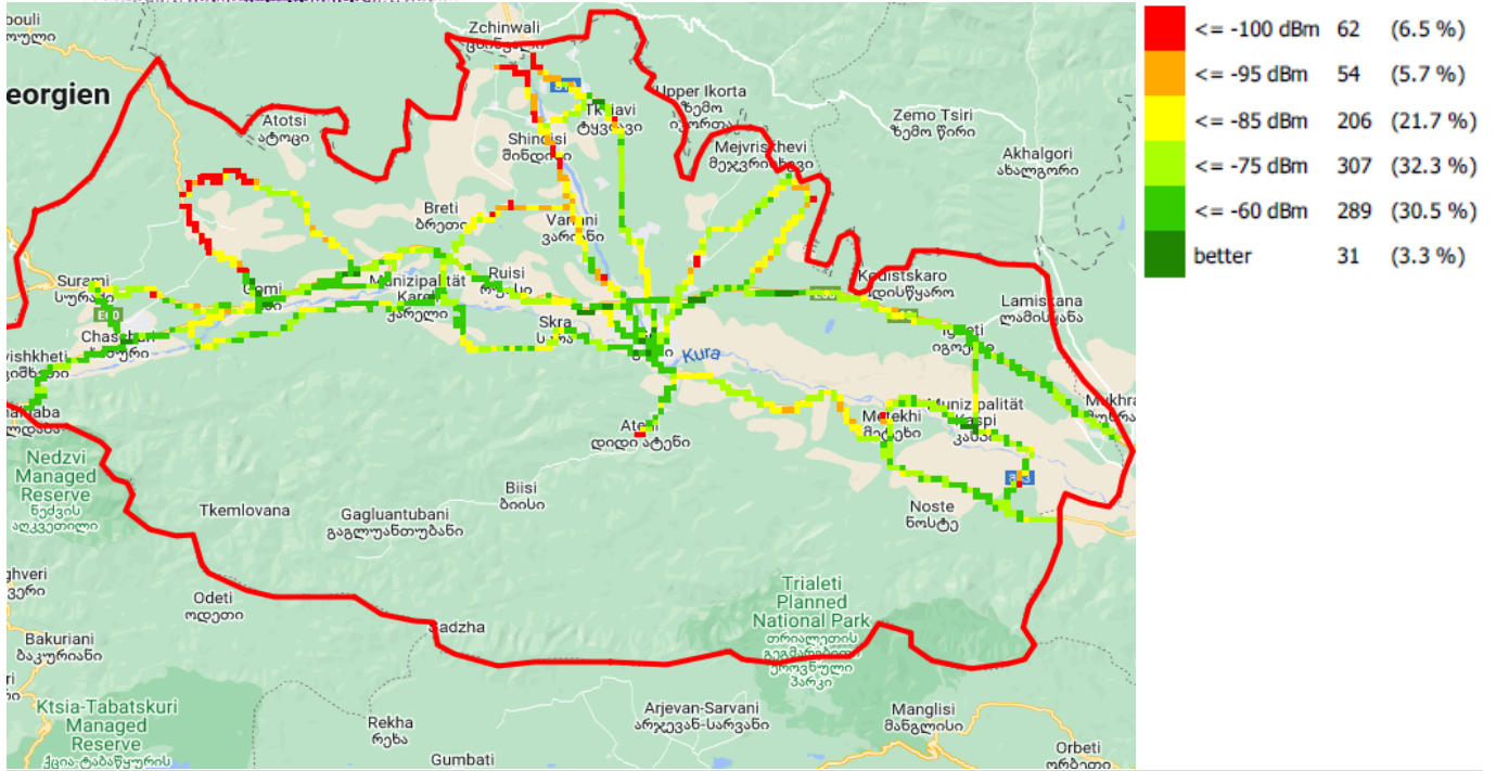
RSCP, ვიონი საქართველო
