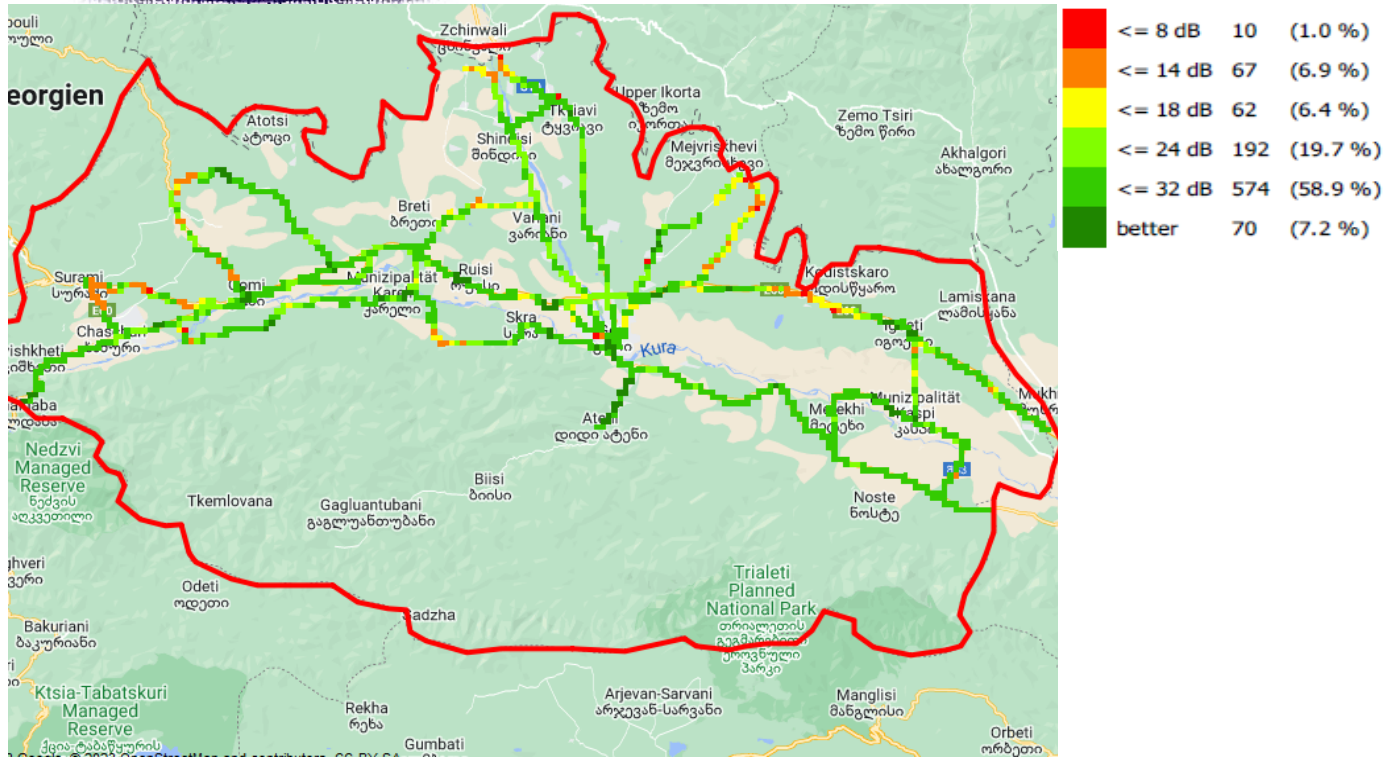
C/I, ვიონი საქართველო
