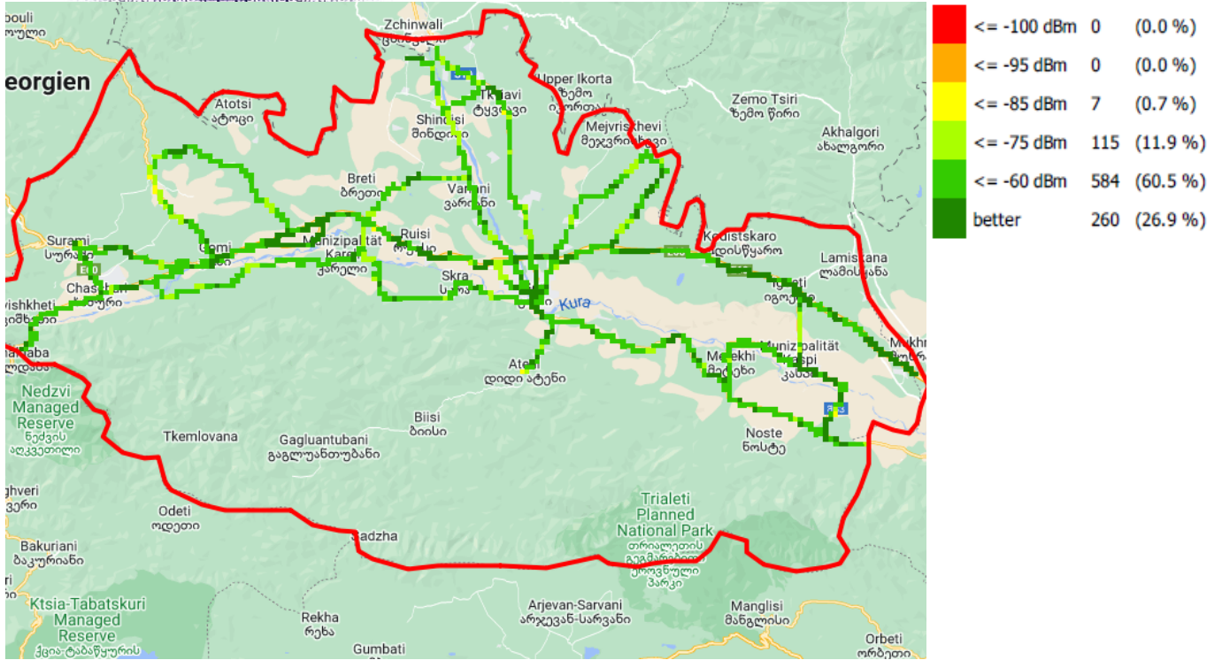
RSCP, მაგთიკომი
