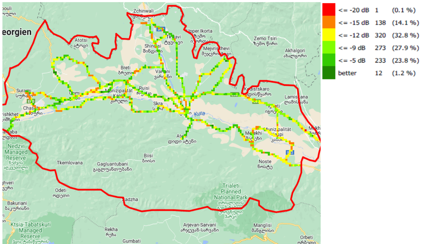
RSRQ, სილქნეტი
