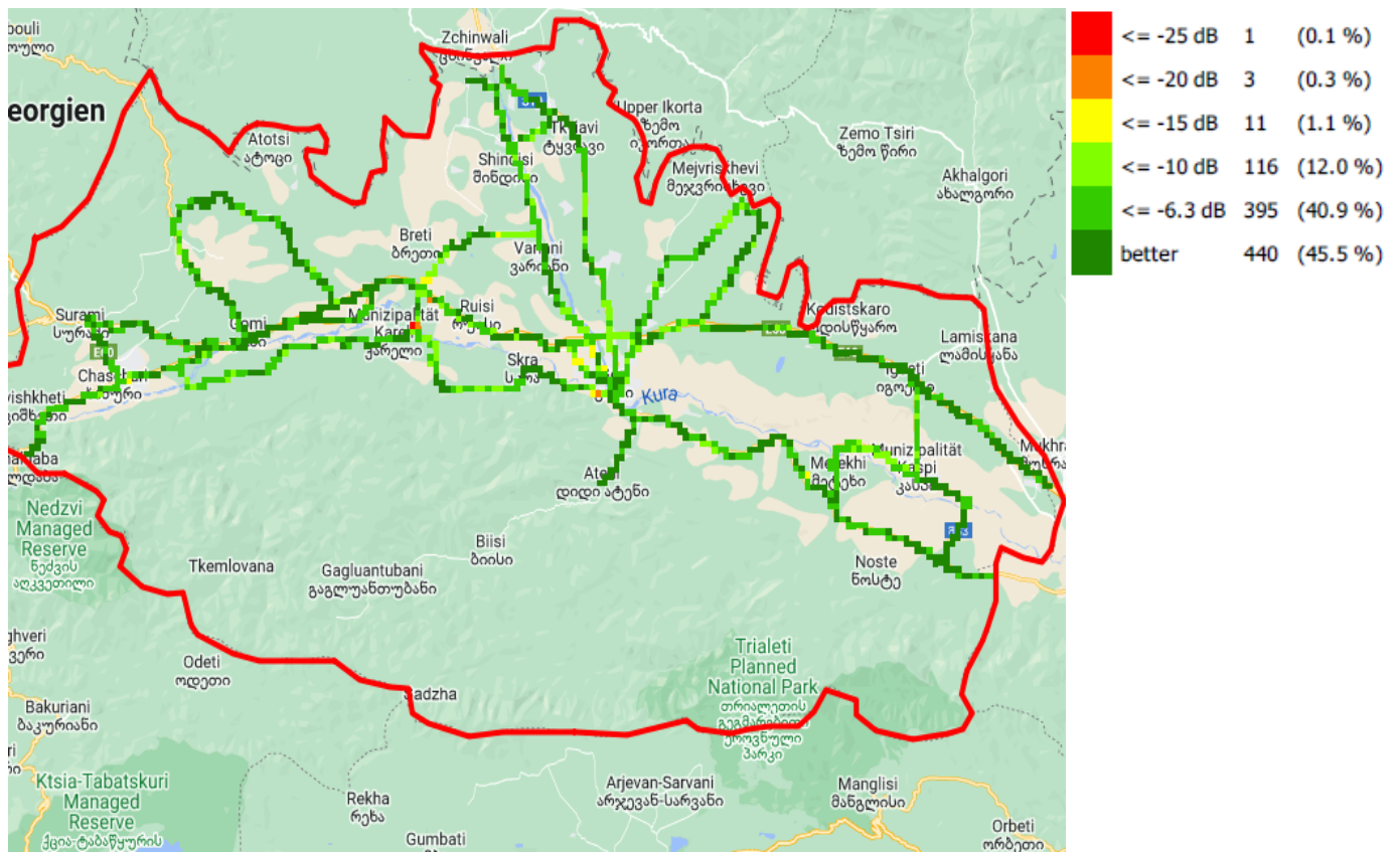
Ec/Io, მაგთიკომი
