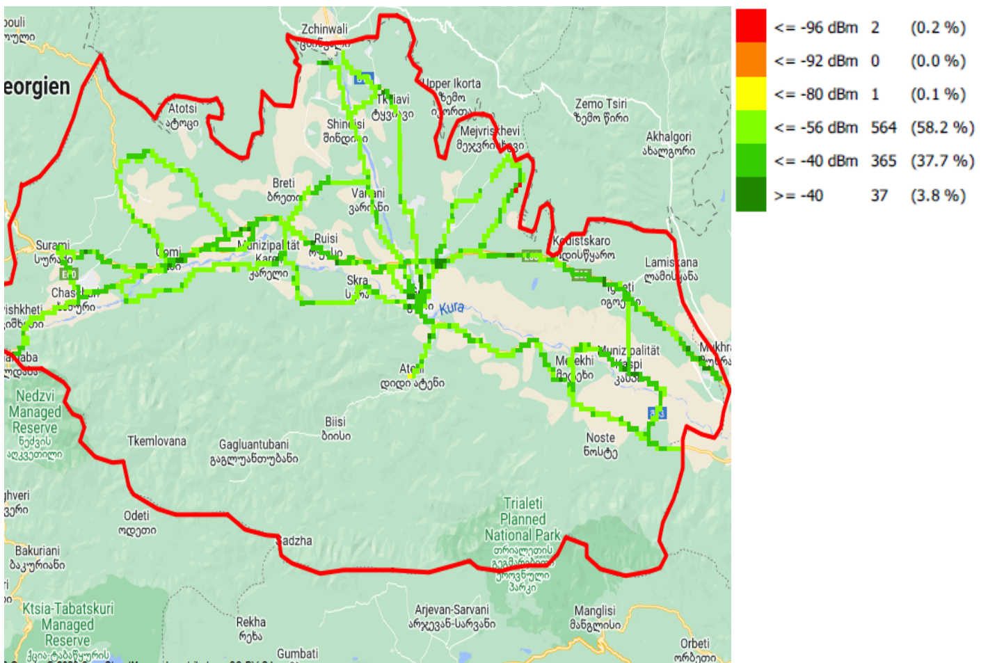
RX_LEV, მაგთიკომი
