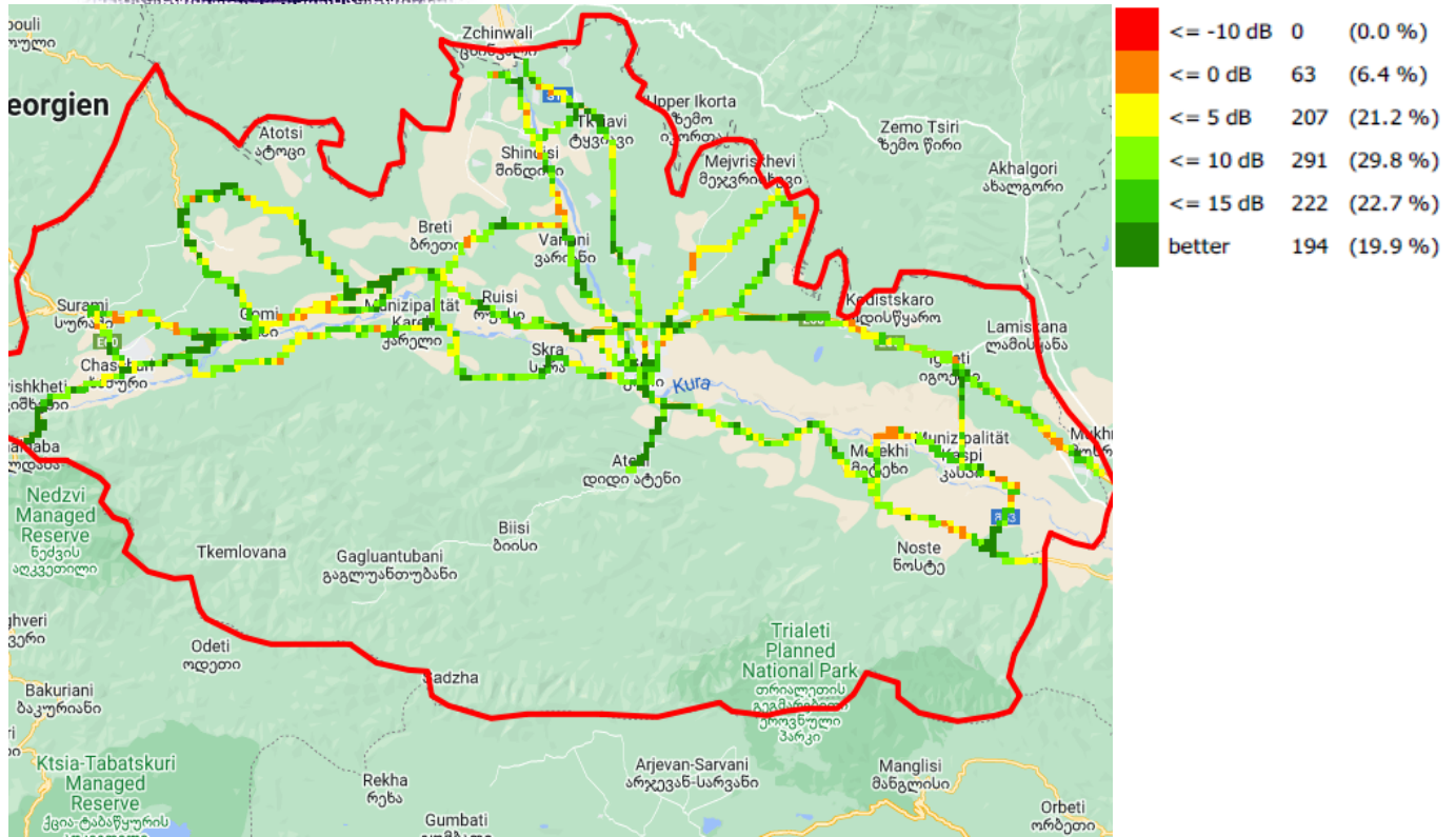
SINR, სილქნეტი
