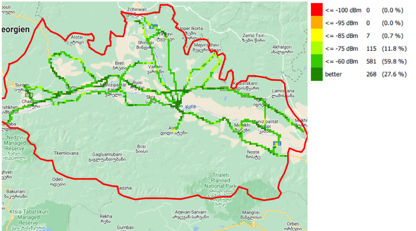
RSCP, სოლენეტი
