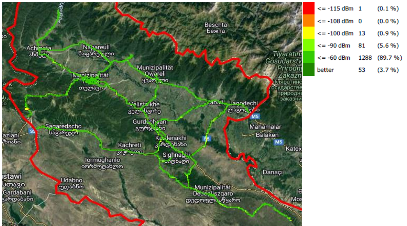
RSRP, მათეოკომი
