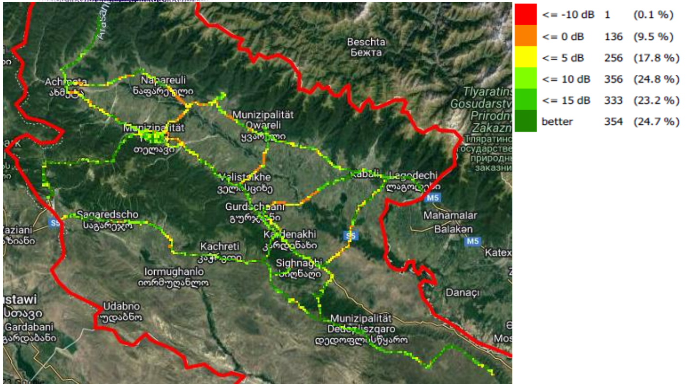
SINR, მგეტიკომი
