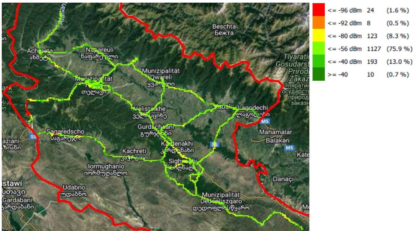
RX_LEV, ვიონი საქართველო
