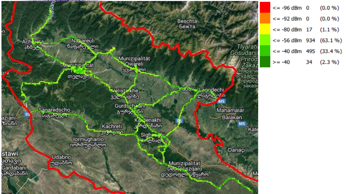
RX_LEV, სილქნეტი
