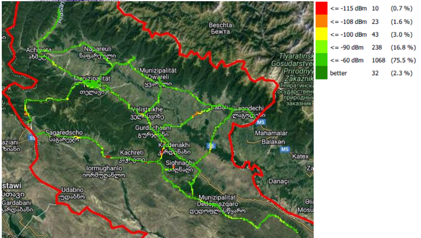
RSRP, ვიონი საქართველო
