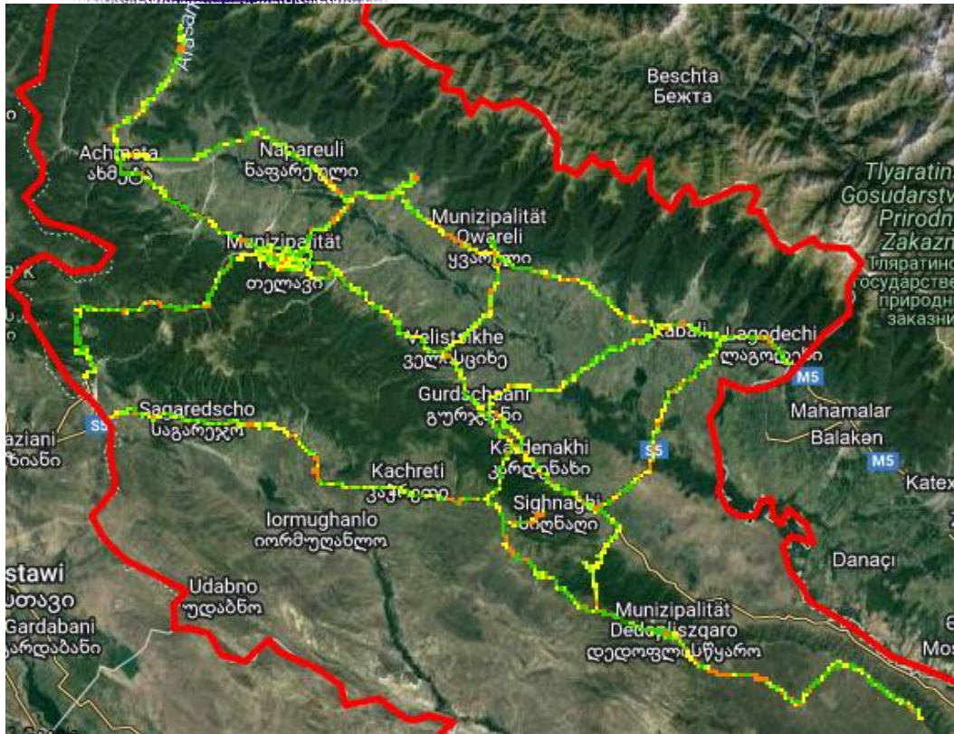
RSRQ სილქნეტი
