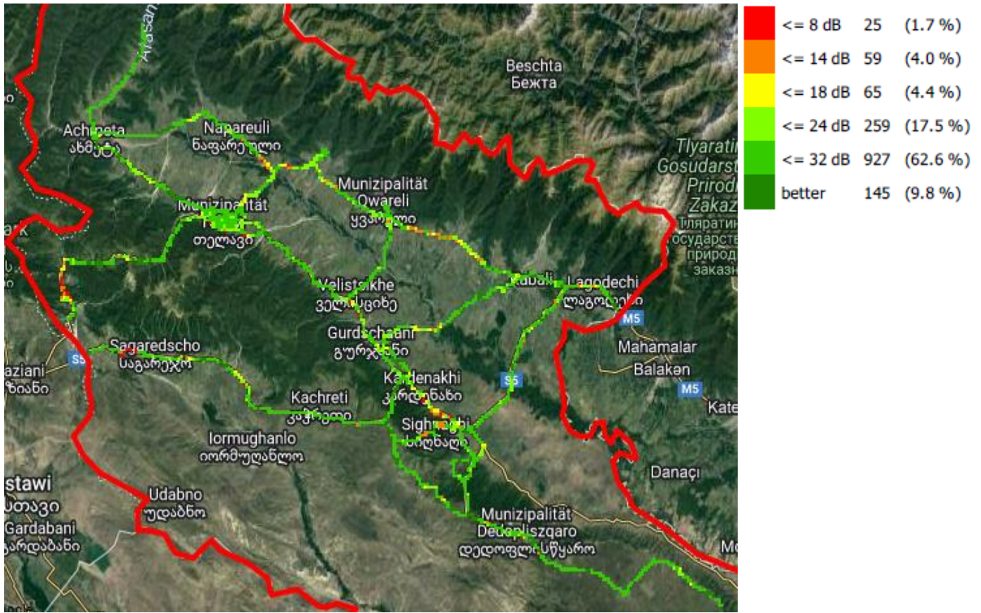
C/I, ვიონი საქართველო
