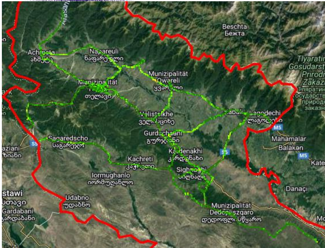
Ec/Io, მაგთიკომი
