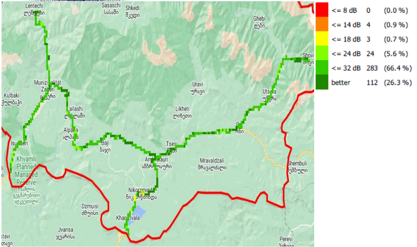
C/I, მაგთიკომი
