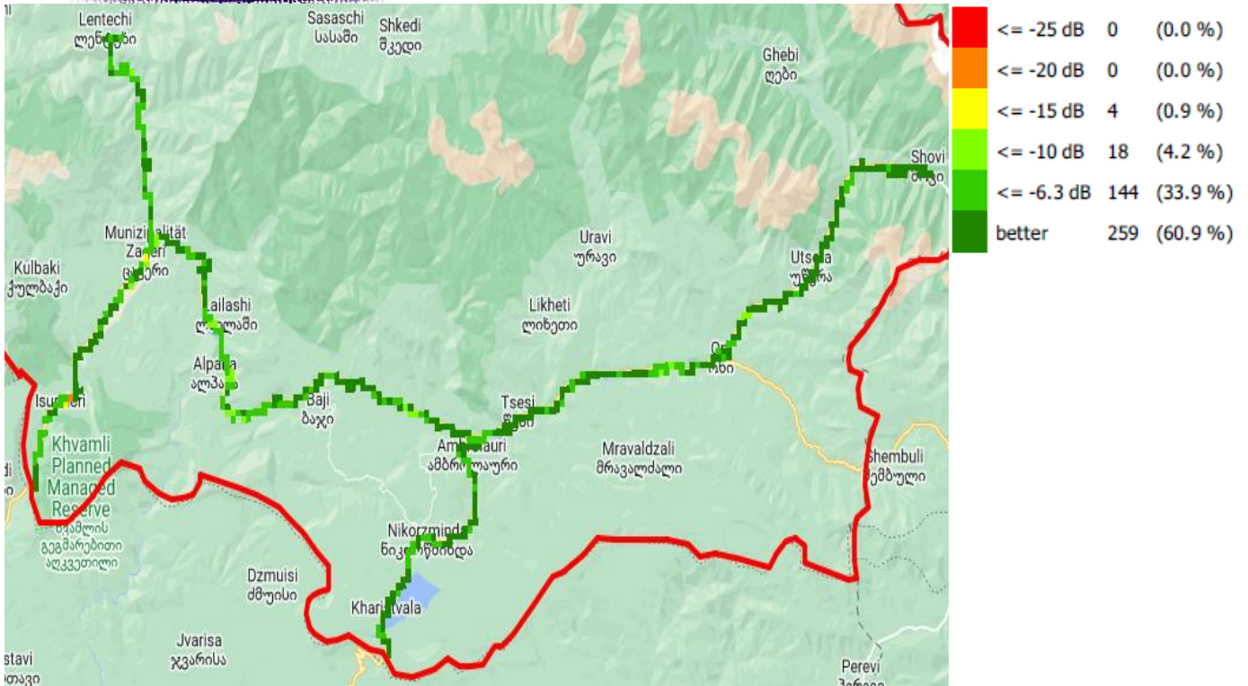
Ec/Io, მაგთიკომი
