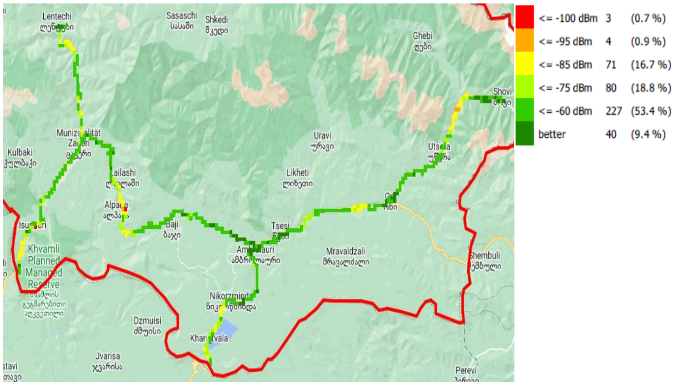
RSCP, მაგთიკომი
