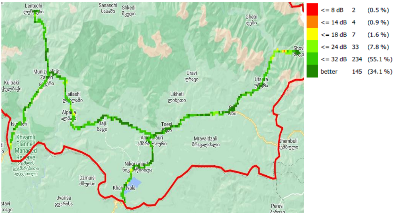
C/I, სილქნეტი
