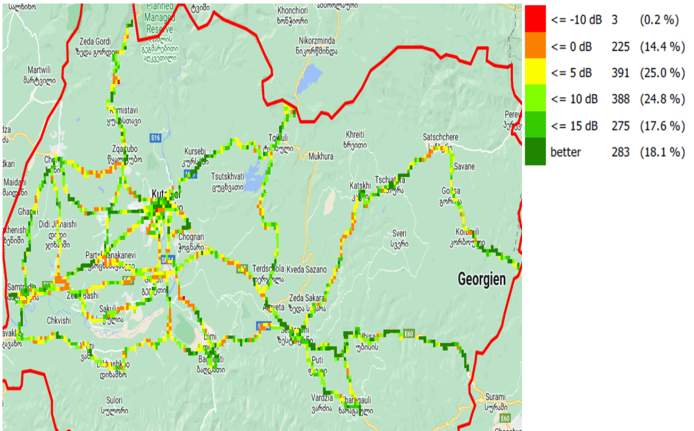
SINA, მაგთიკომი
