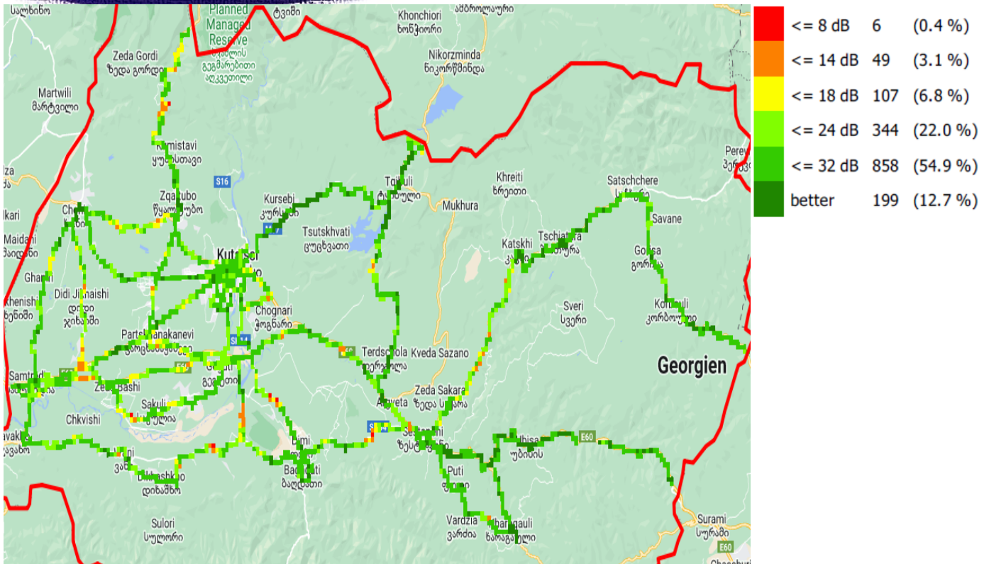
C/I, მატეიკომი
