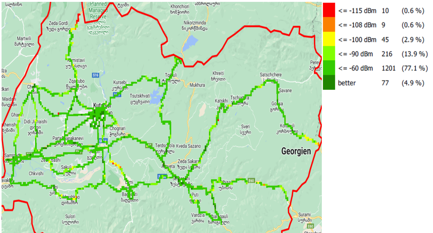
RSRP, სოლენეტი
