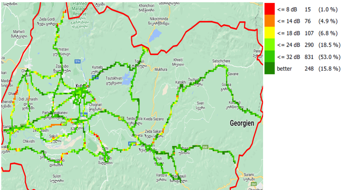
C/I, სილქნეტი
