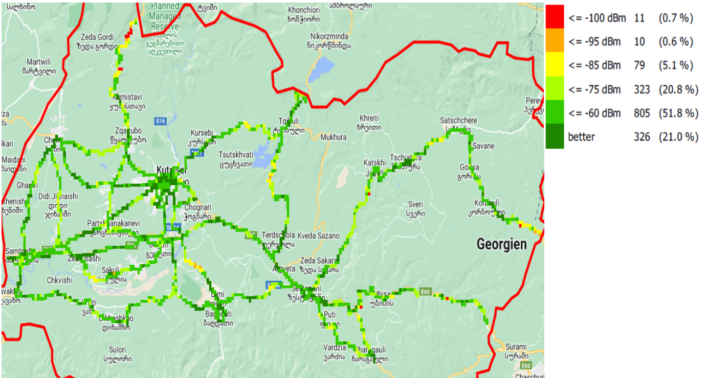
RSCP, მატეიკომი
