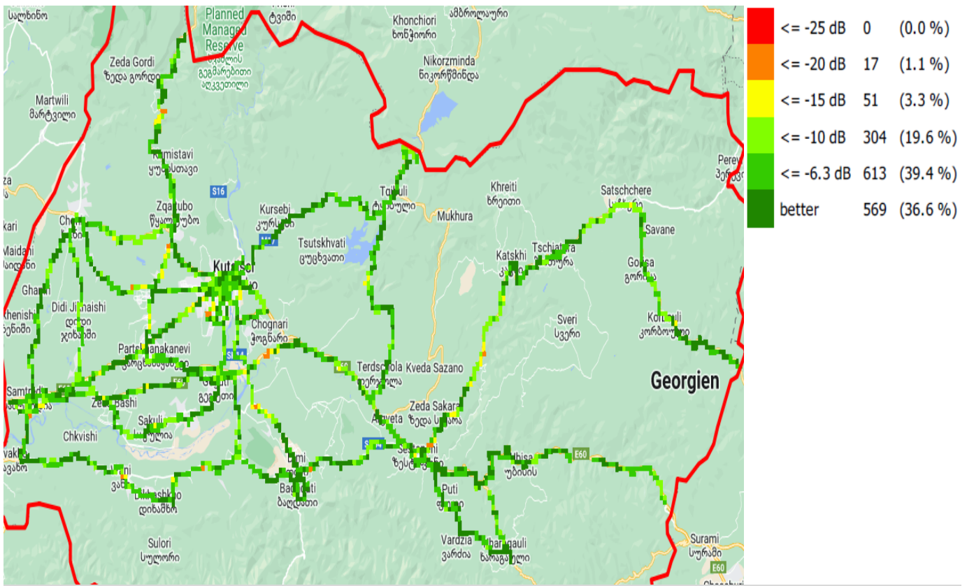
Ec/Io, მაგთიკომი
