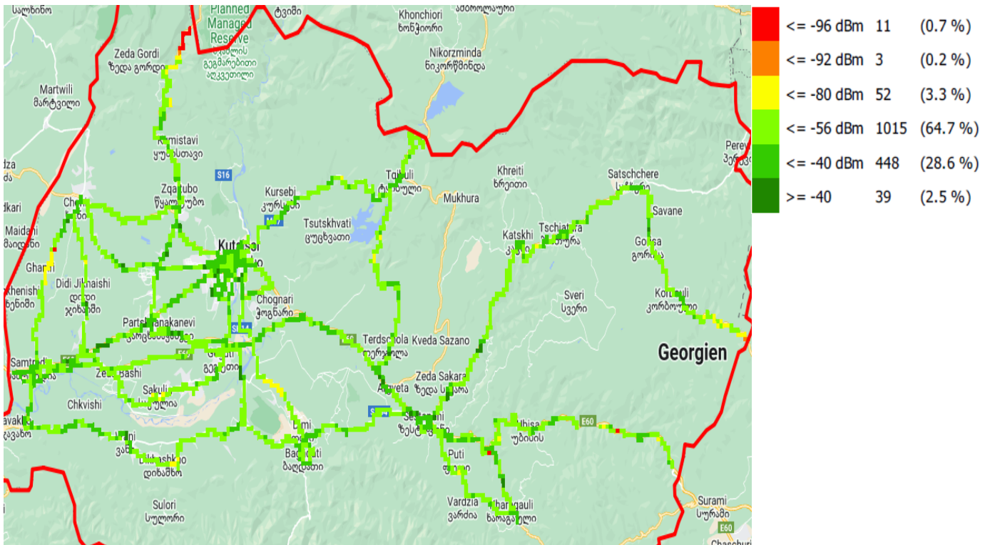
RX_LEV, სილქნეტი
