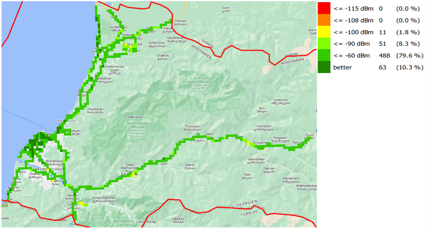
RSRP, მათეკომი
