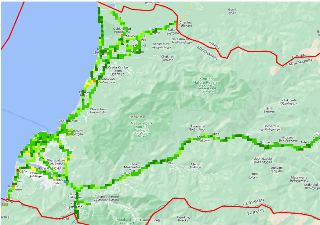
Ec/Io, სილქნეტი
