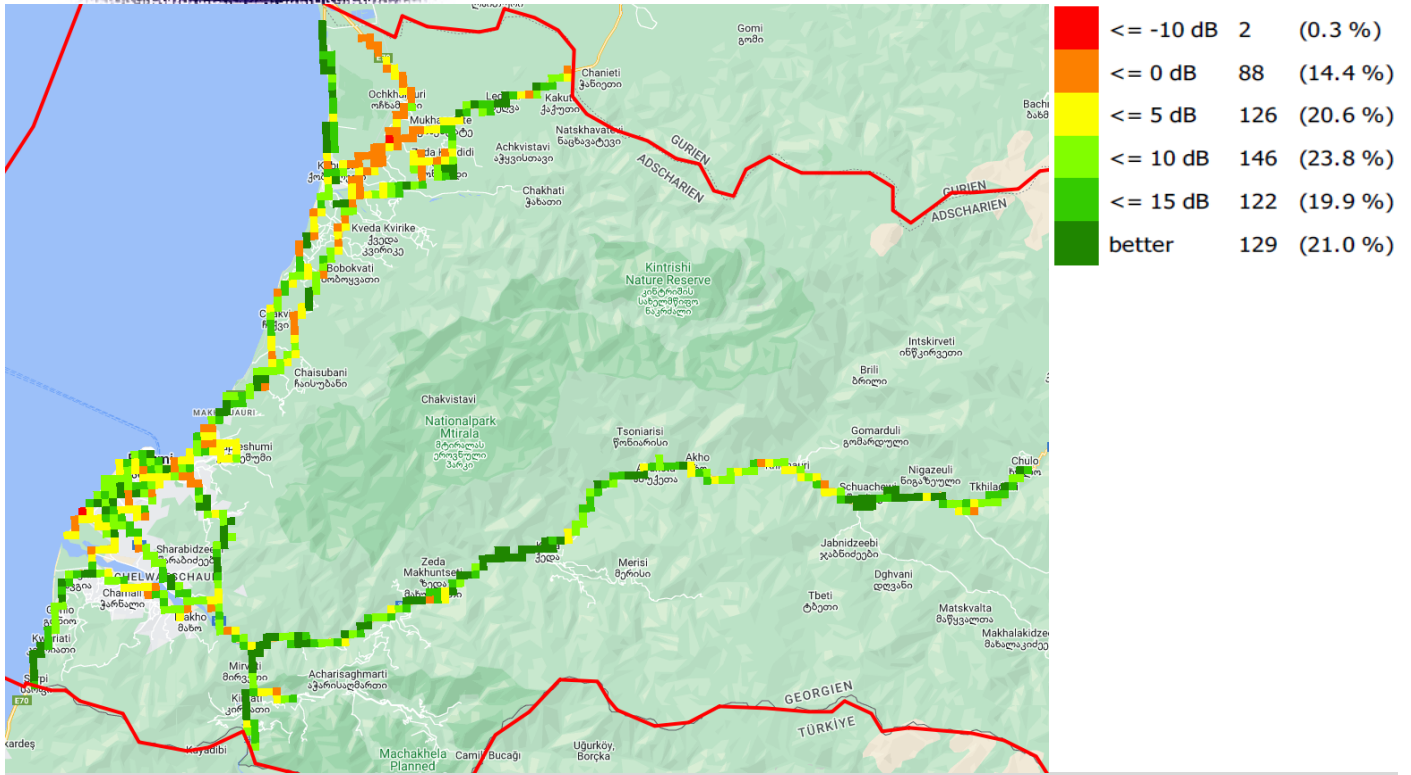
SINR, მათეოკომი
