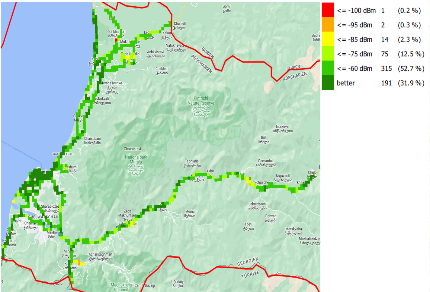
RSCP, მაგთიკომი
