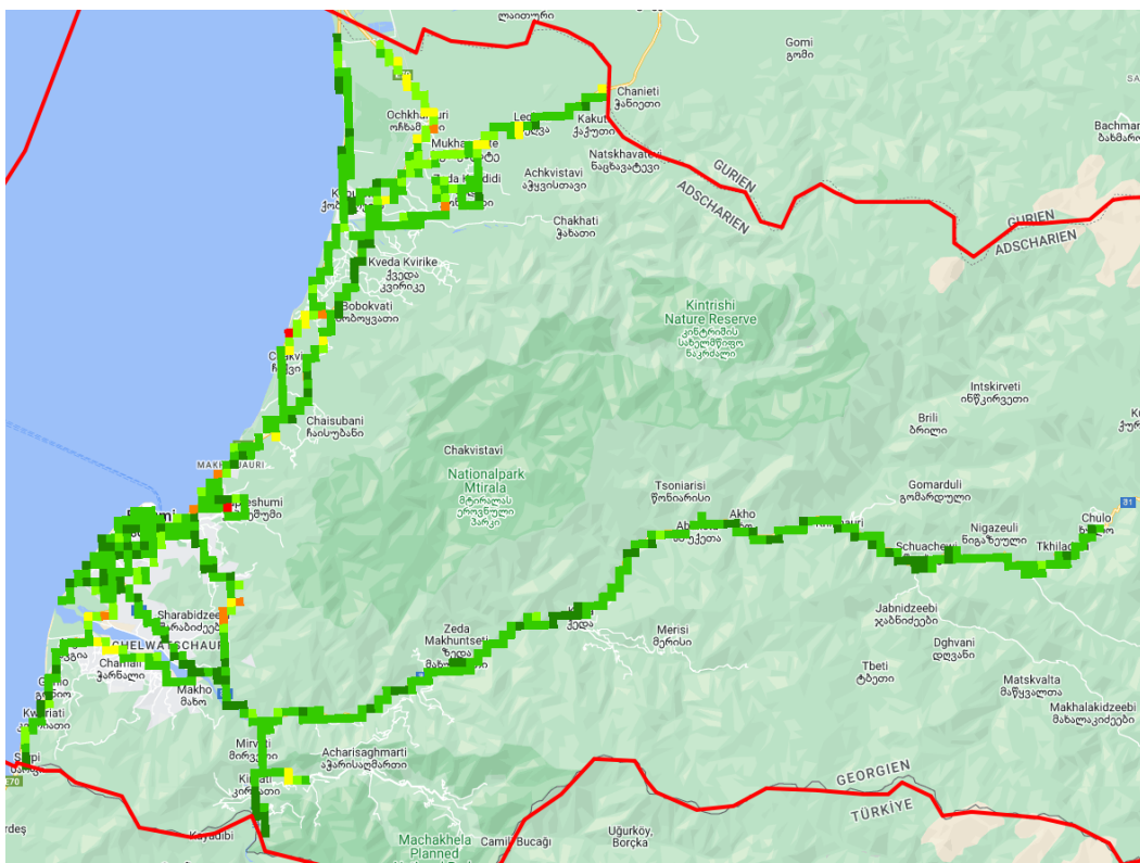
C/I, სოლქნეტი
