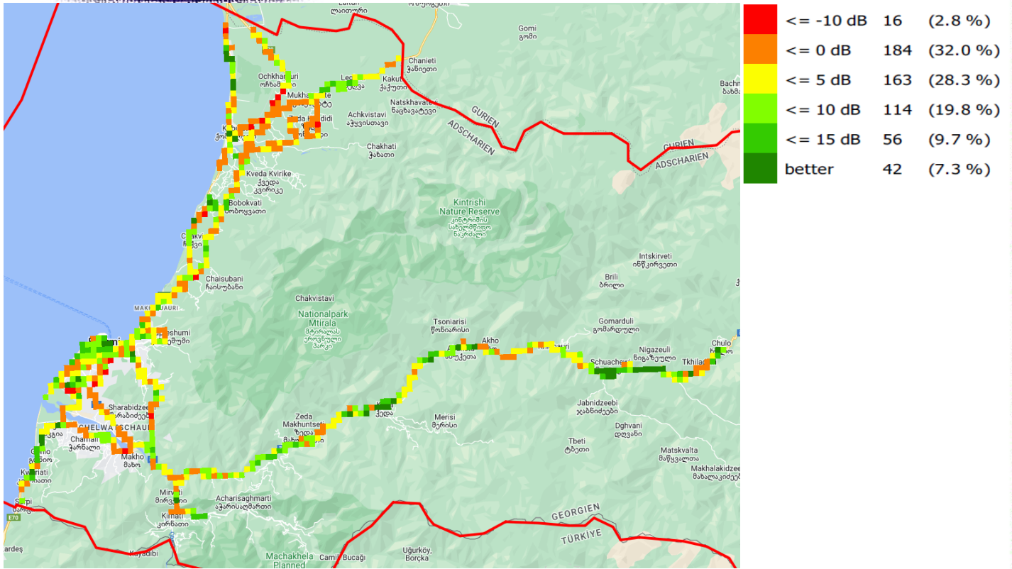
SINR, სელგი
