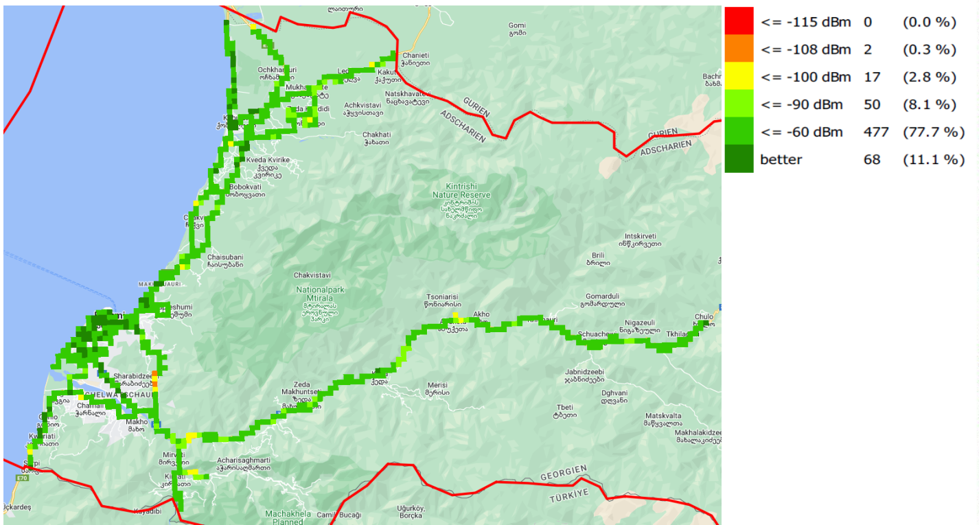
RSRP, სილქნეტი
