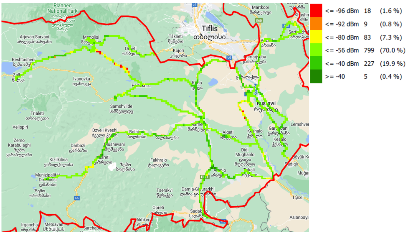
RX_LEV, სელცი
