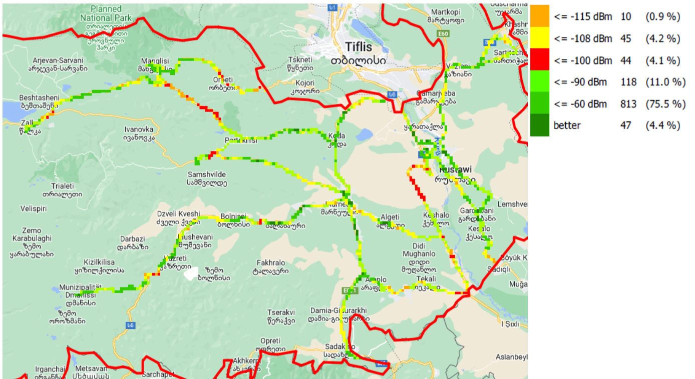
RSCP, სელვი
