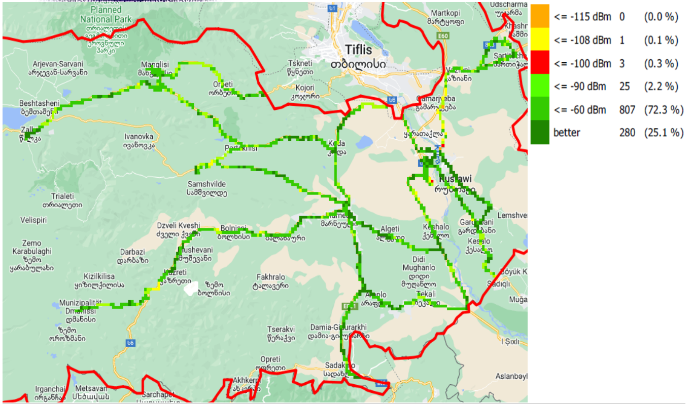
RSCP, სოლნეტი
