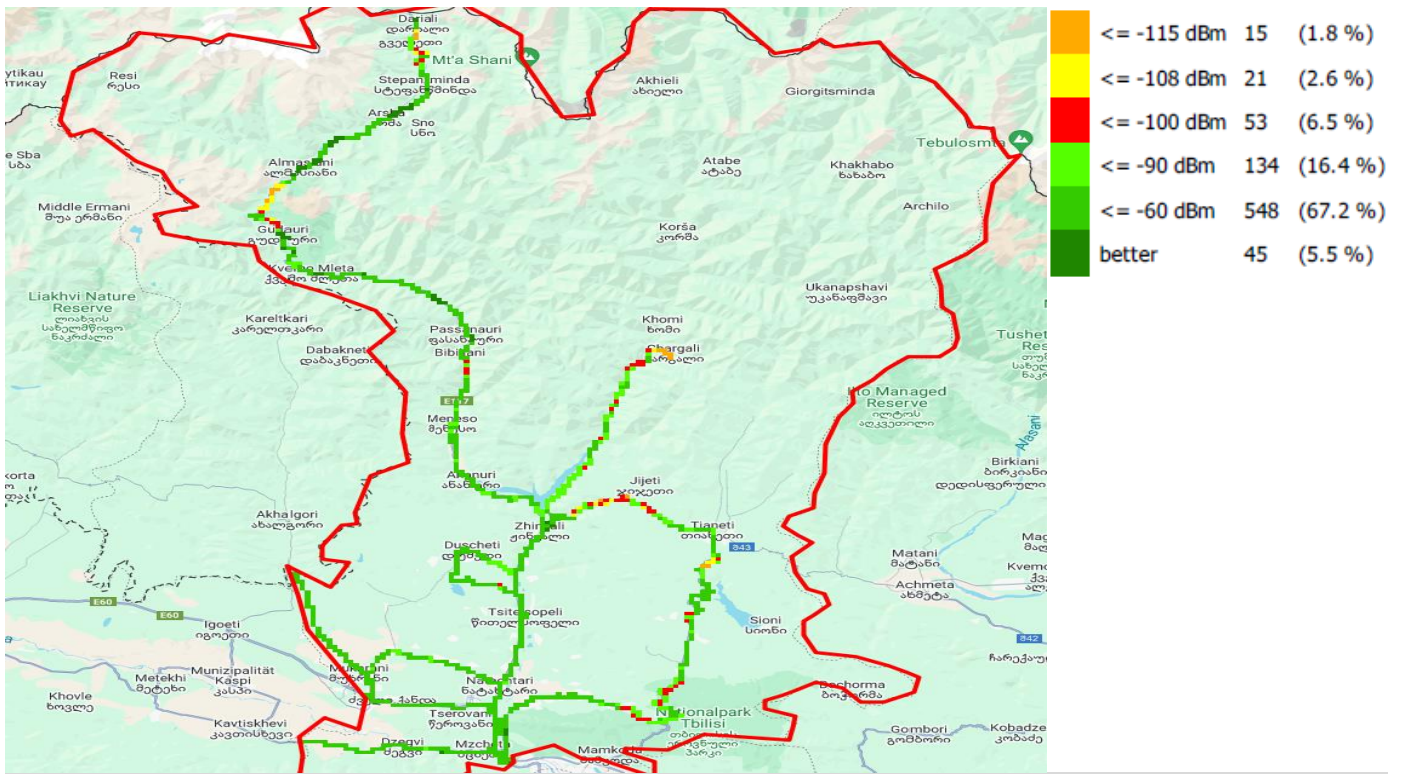
RSCP, სელგე
