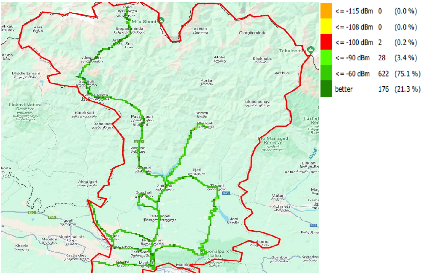
RSCP, მაგთიკომი
