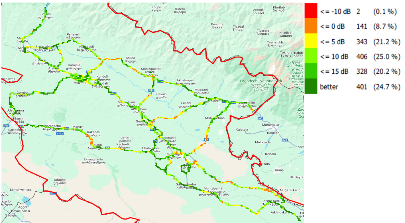
SINR, სილქნეტი
