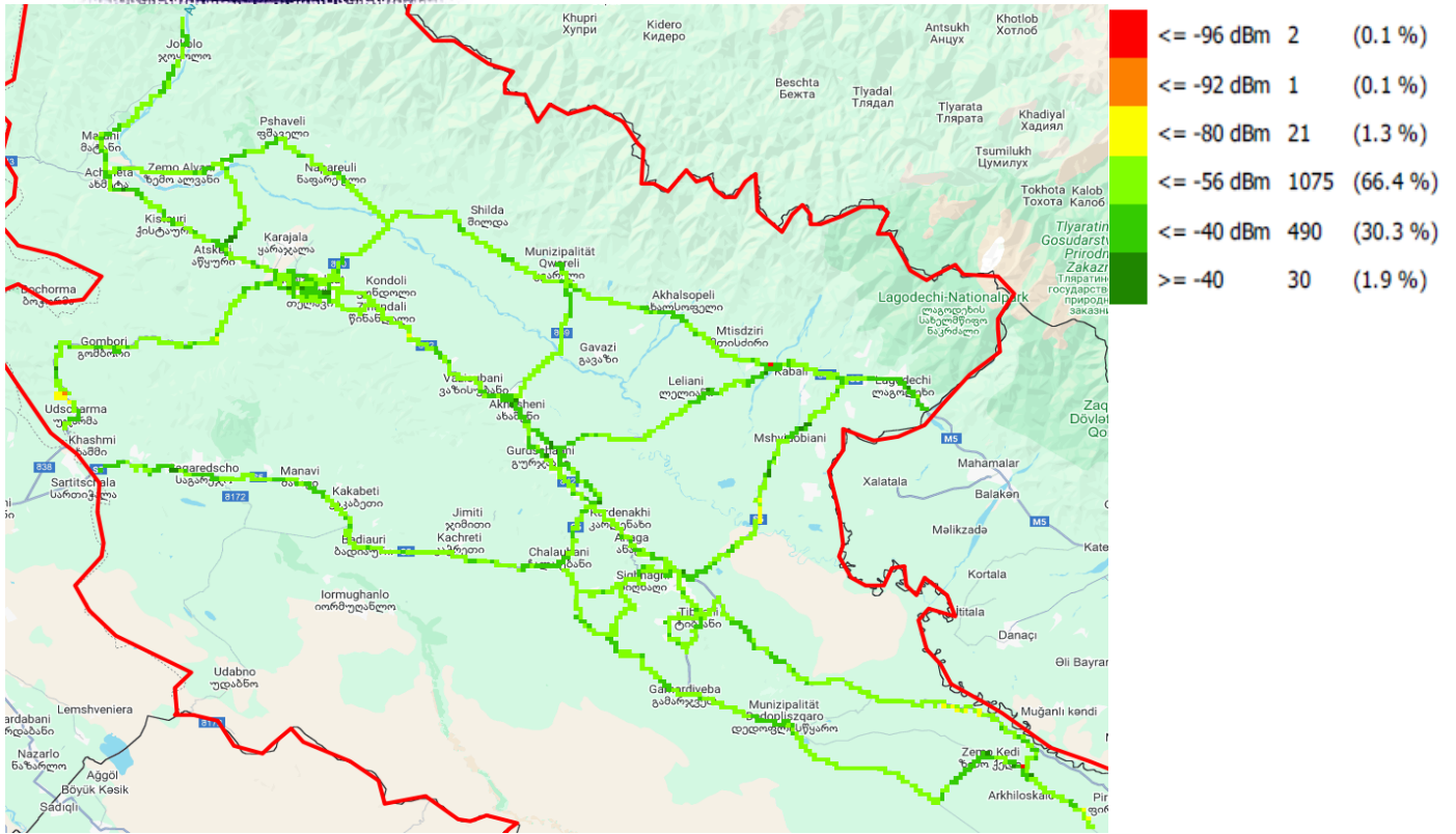
RX_LEV, მაგთიკომი
