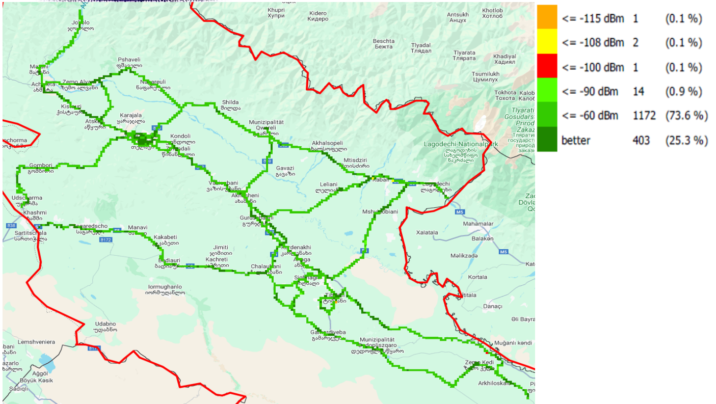
RSCP, სილქნეტი
