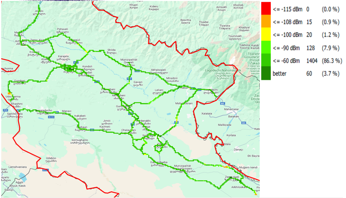
RSRP, მავთიკომი
