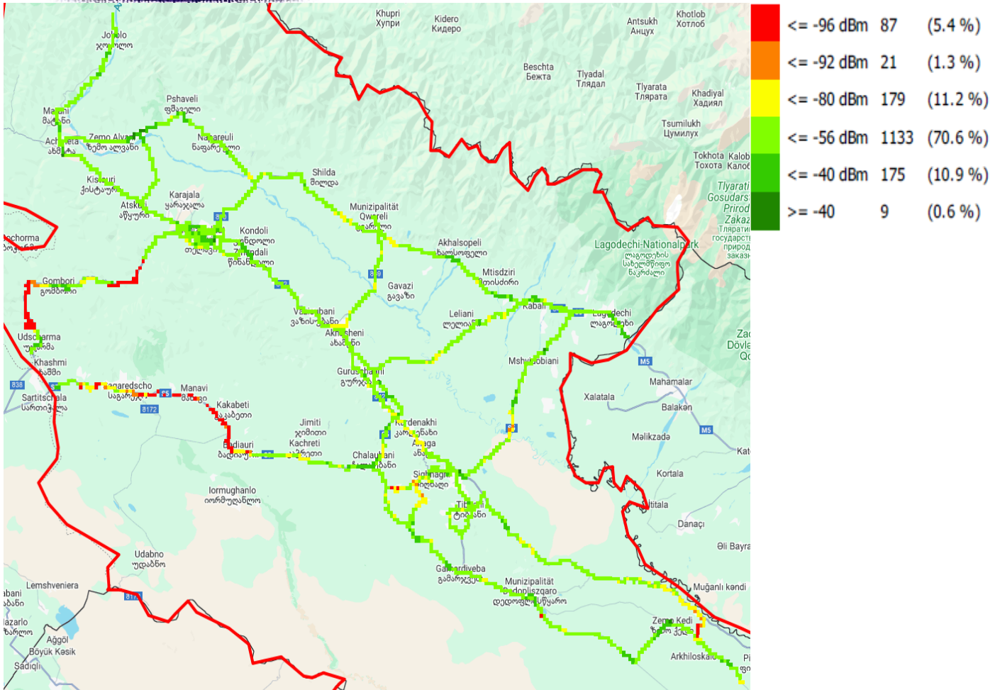
RX_LEV, სელფი
