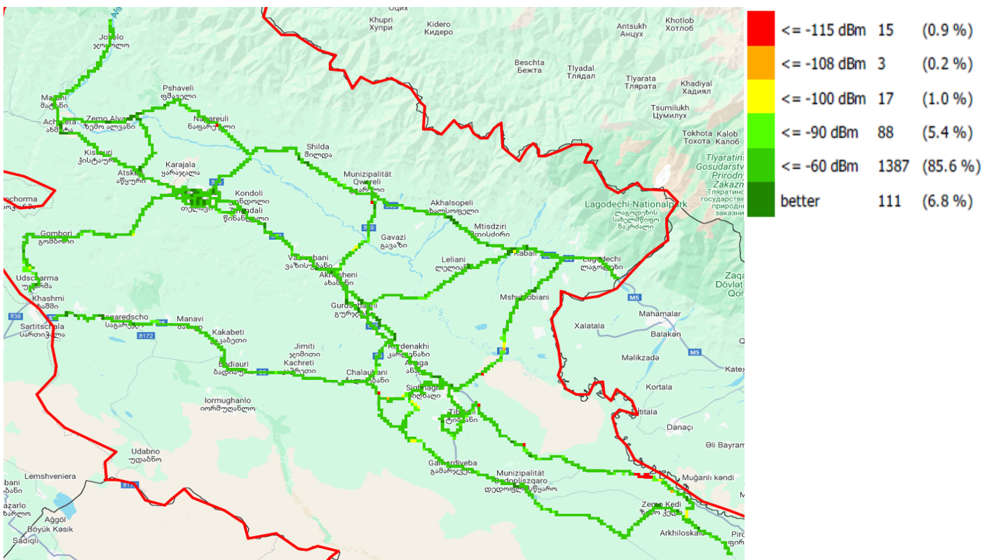
RSRP, სილენეტი
