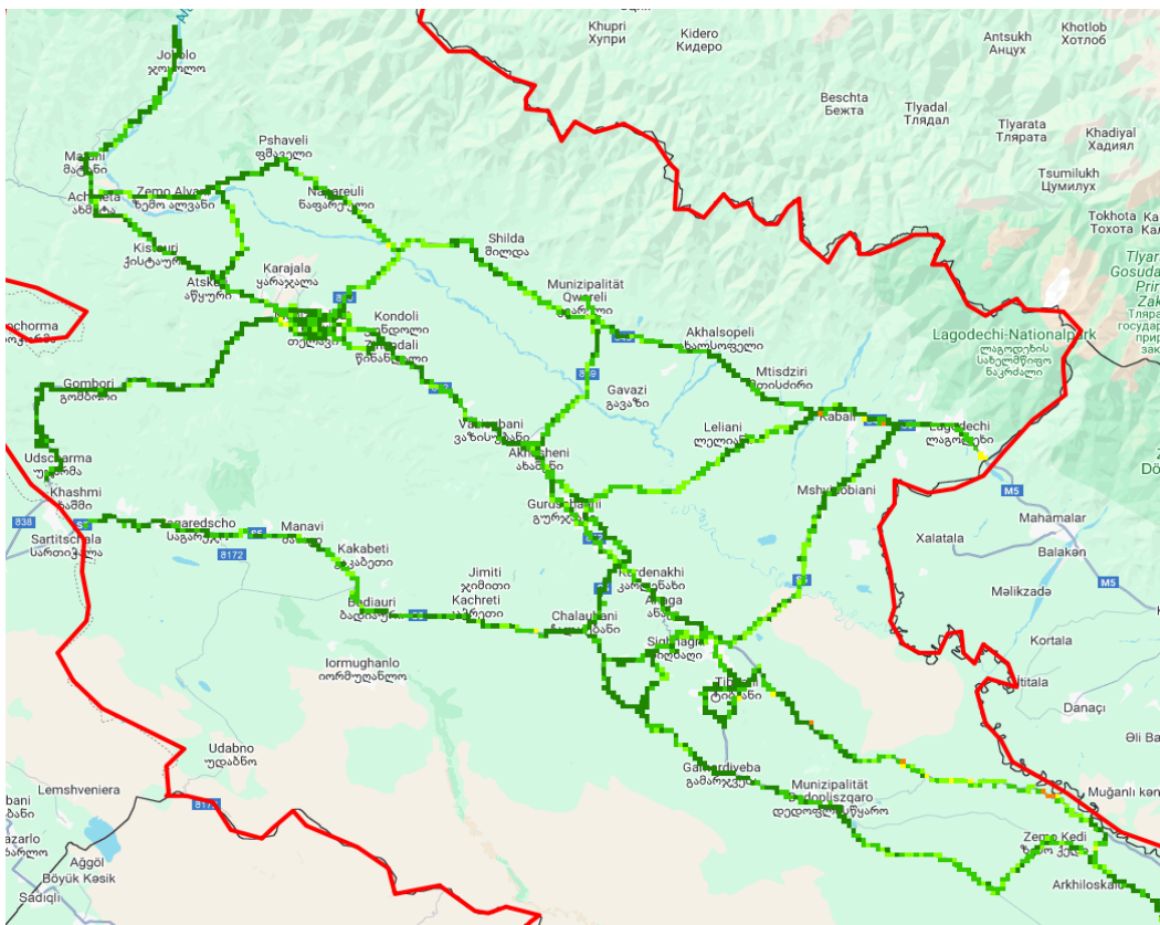
Ec/Io, სოლქნეტი
