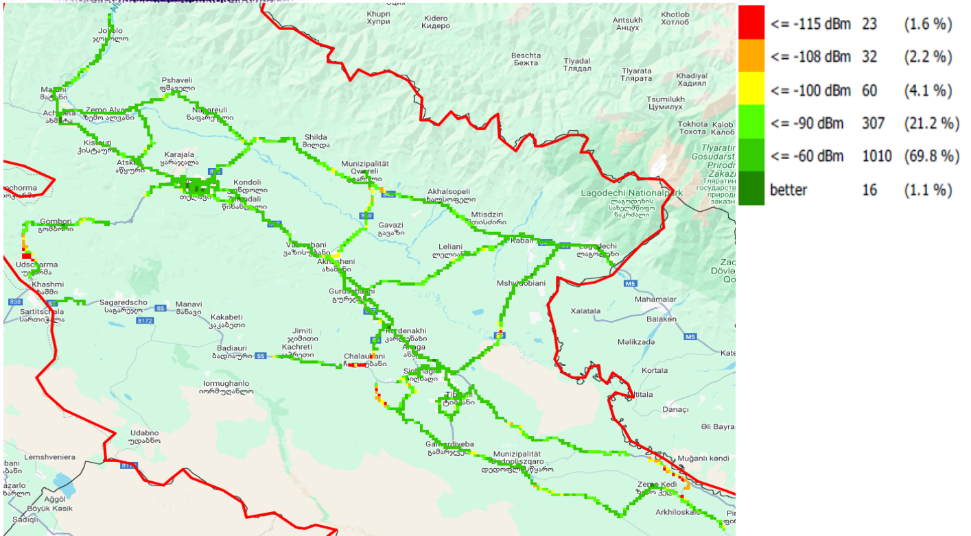
RSRP, სეგვი
