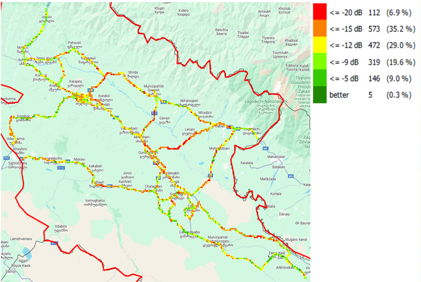
RSRQ, მაგთიკომი
