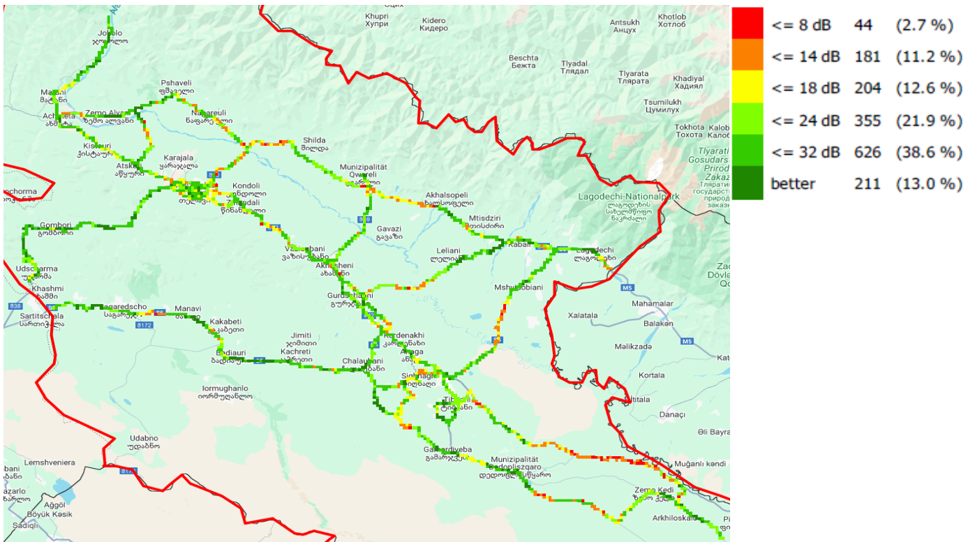
C/I, სოლქნეტი
