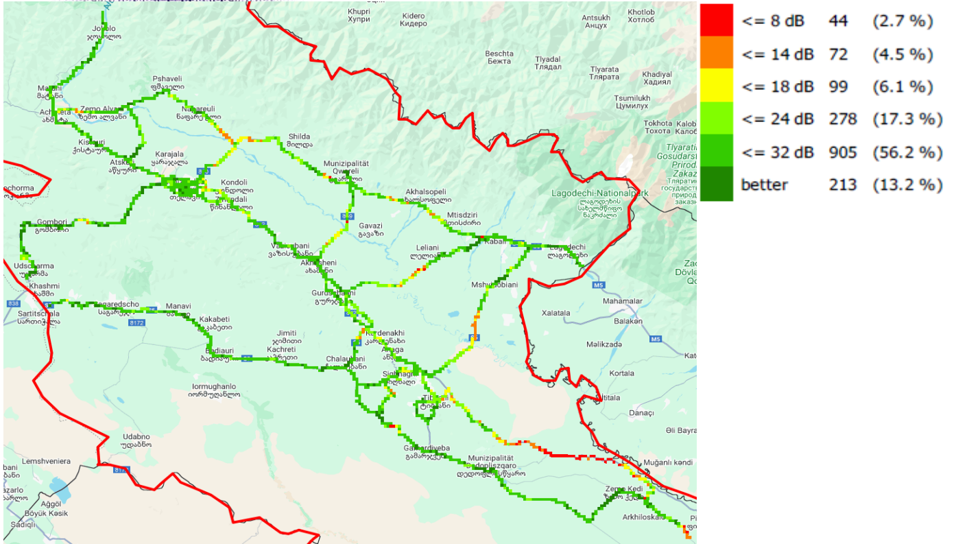
C/I, მათეოკომი
