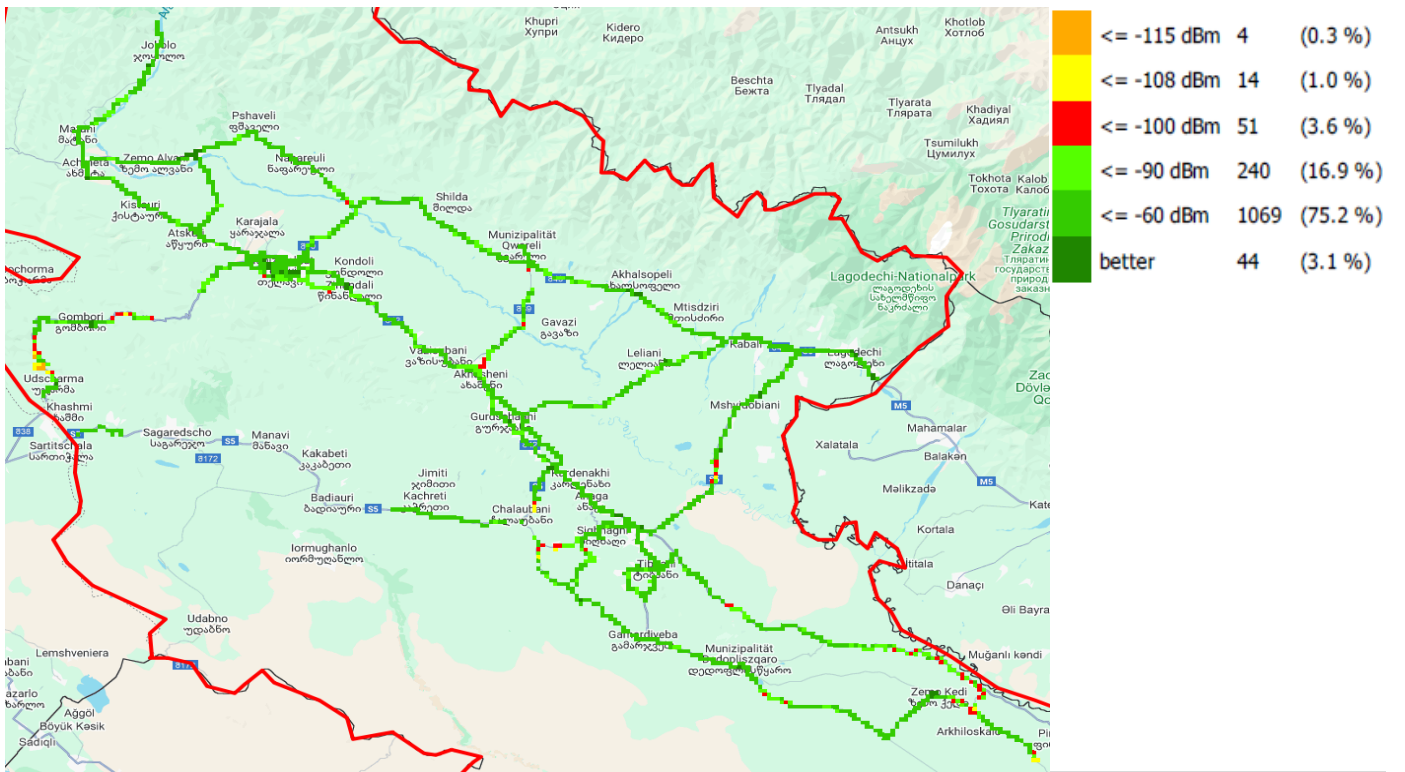
RSCP, სელგეი
