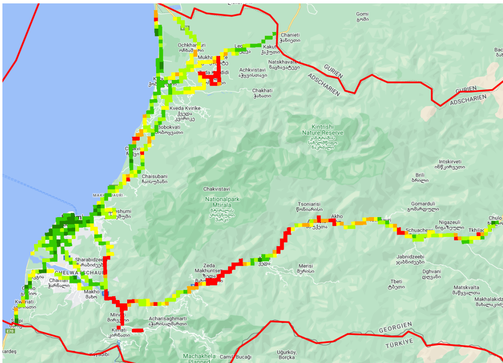
RSCP, სელგო
