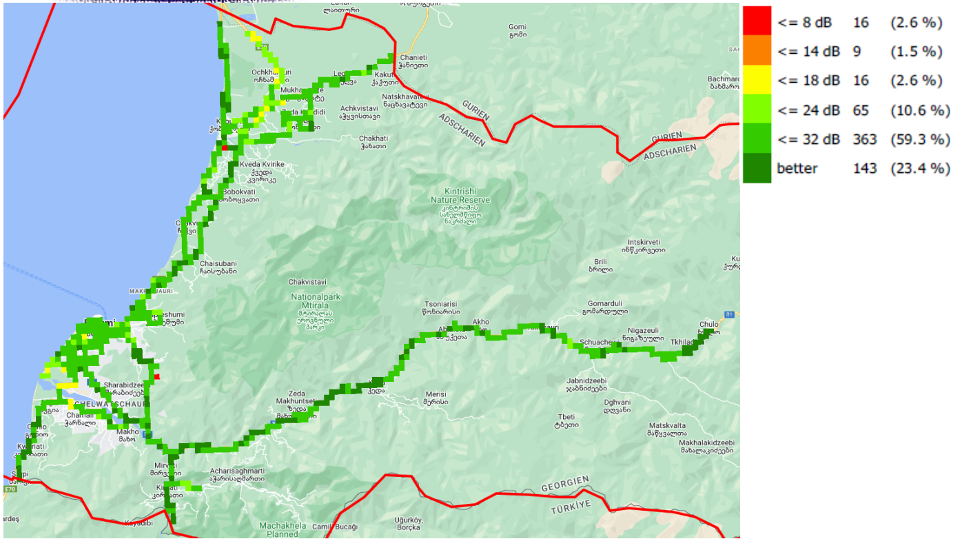
C/I, მათეოკომი
