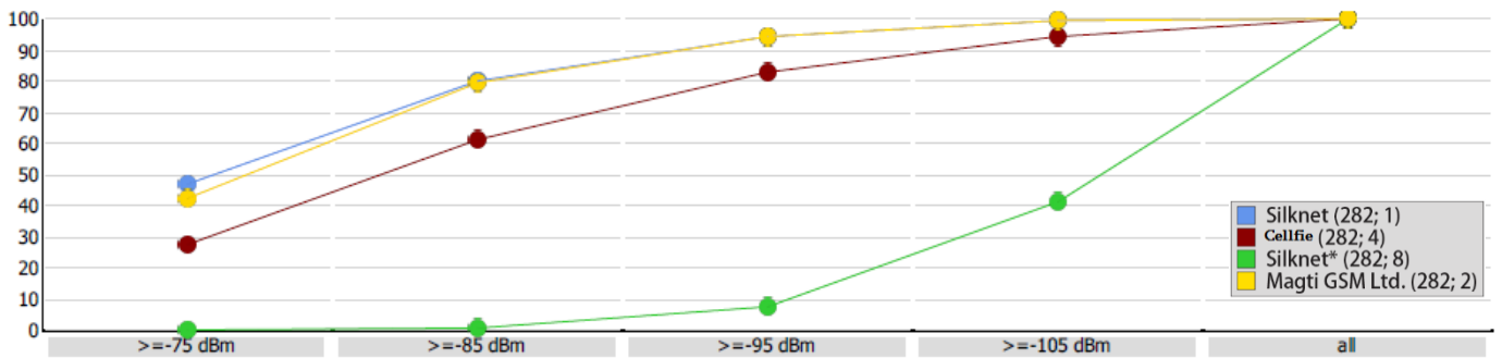
RSRP, სელფი
