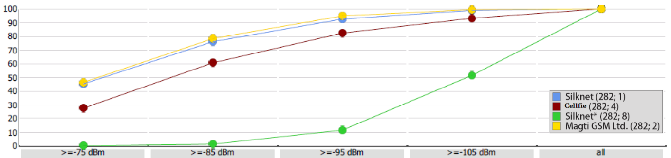
RSRP, სელგი
