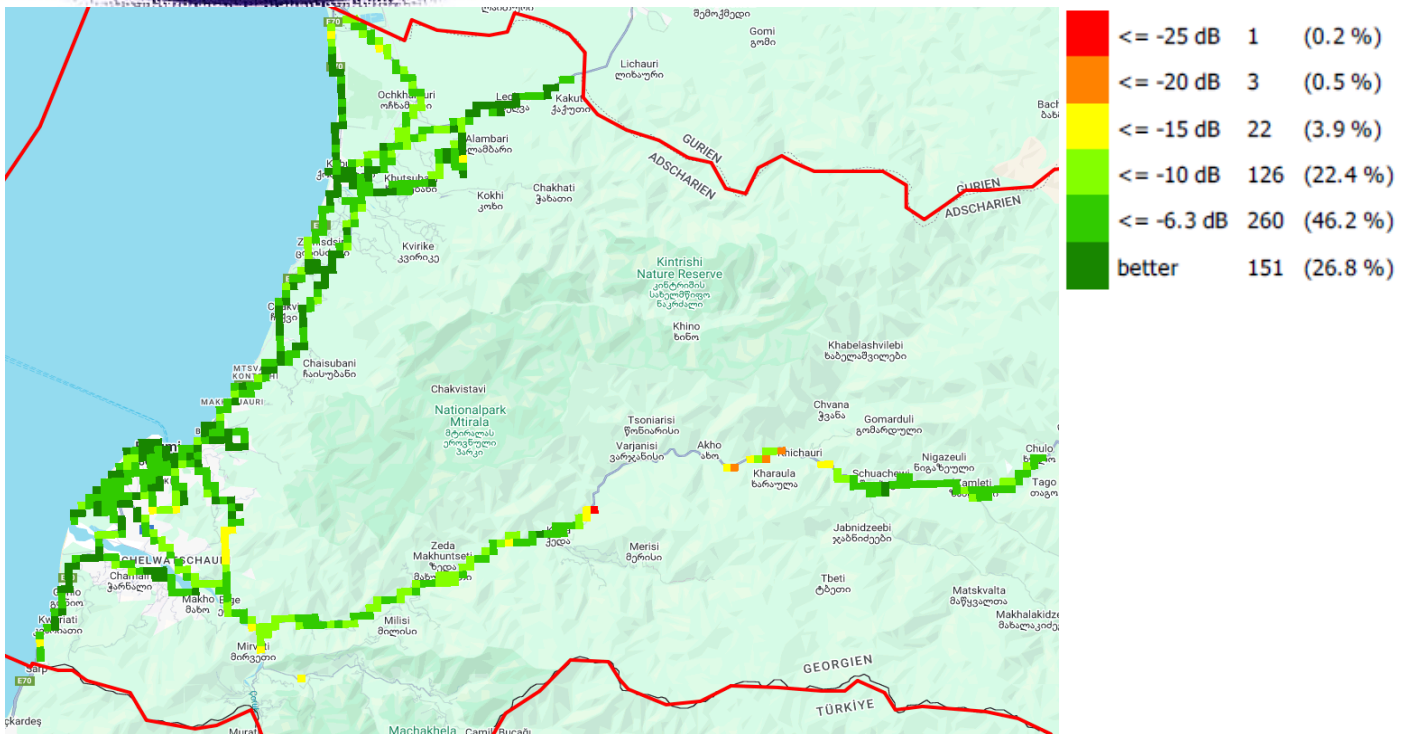
Ec/Io, სელები
