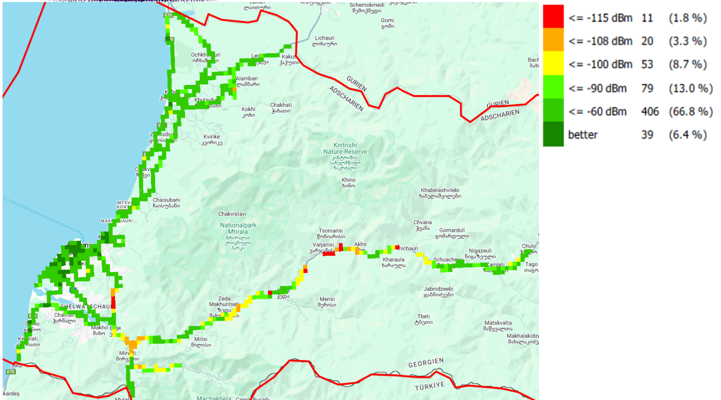
RSRP, სელგი
