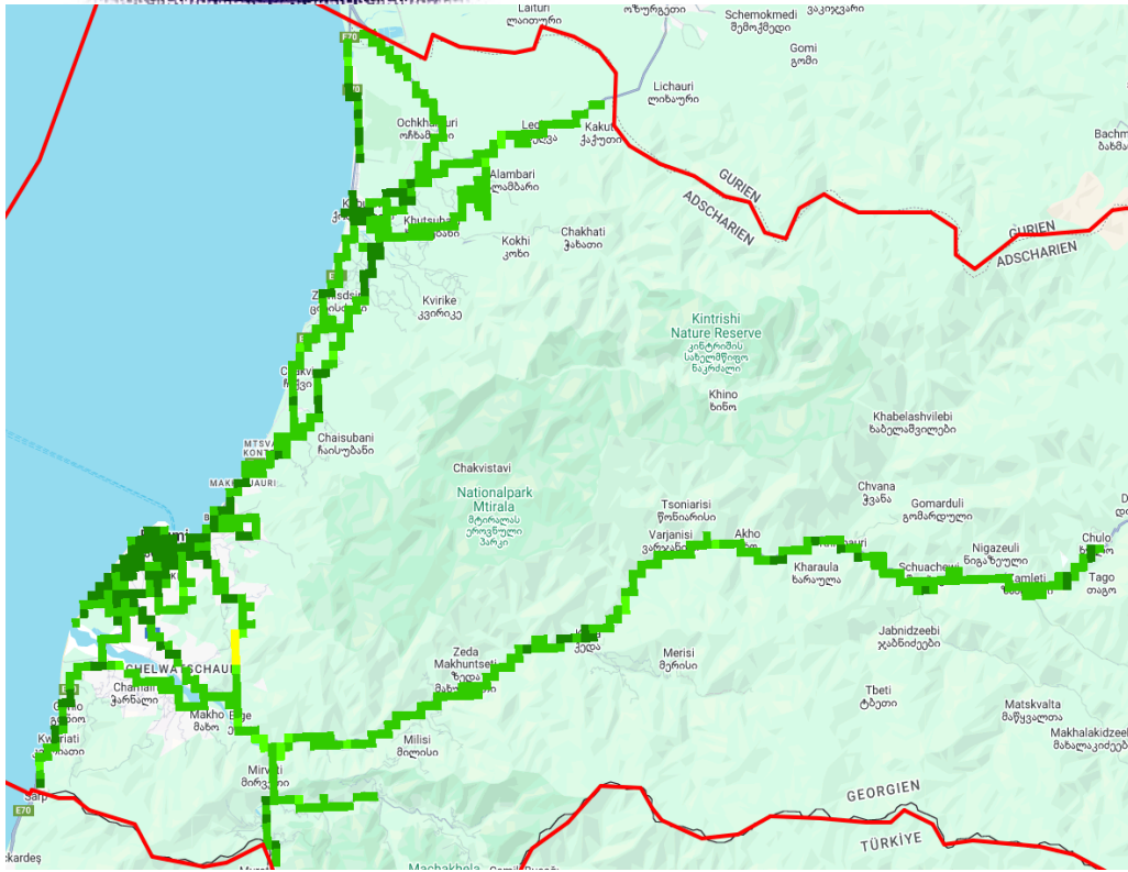
RSCP, სილქნეტი
