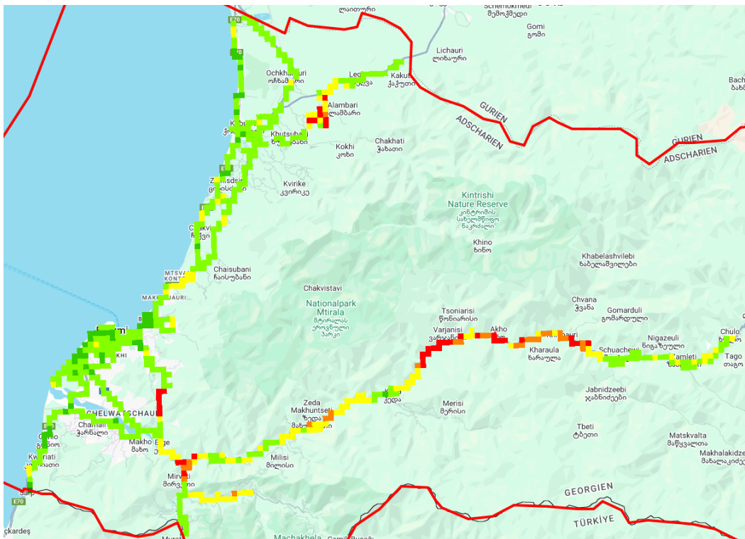
RX_LEV, სელი
