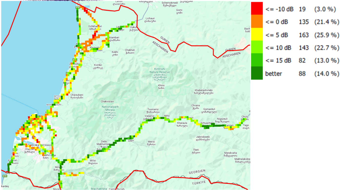
SINR, მაგთიკომი
