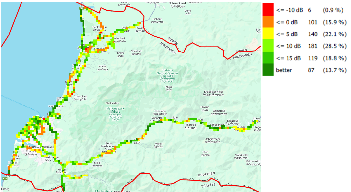
SINR, სილქნეტი
