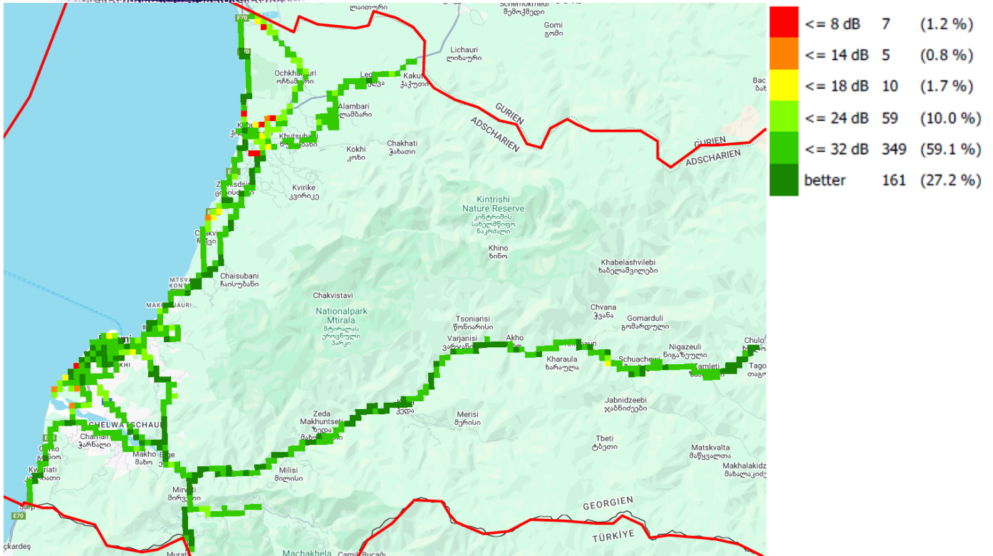
C/I, მაგთიკომი
