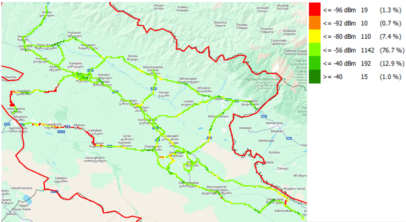
RX_LEV, სელფი
