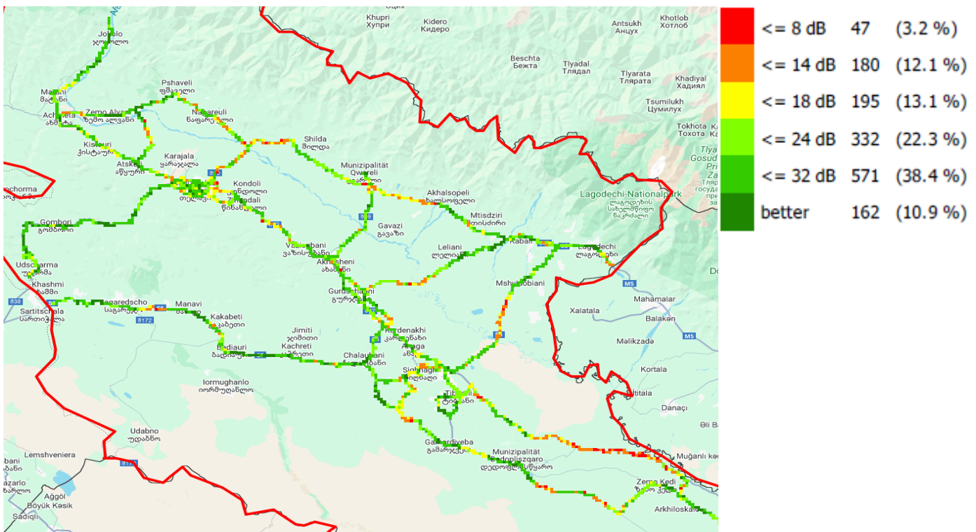
C/I, სილქნეტი
