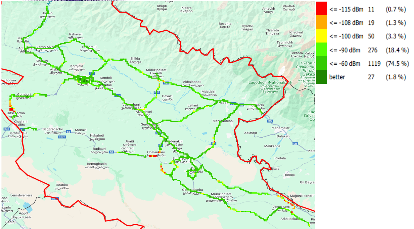
RSRP, სელო
