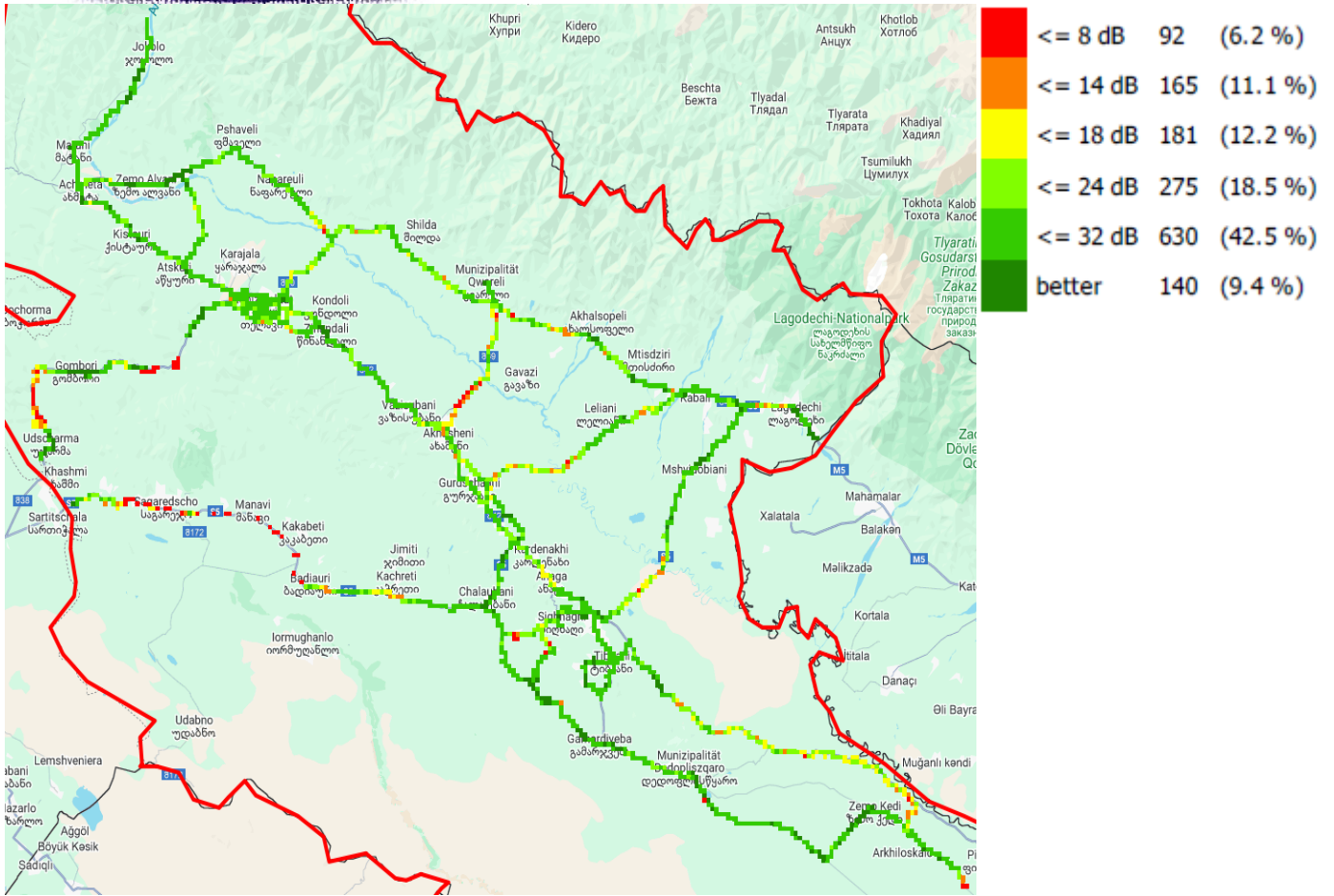
C/I, სეღვი
