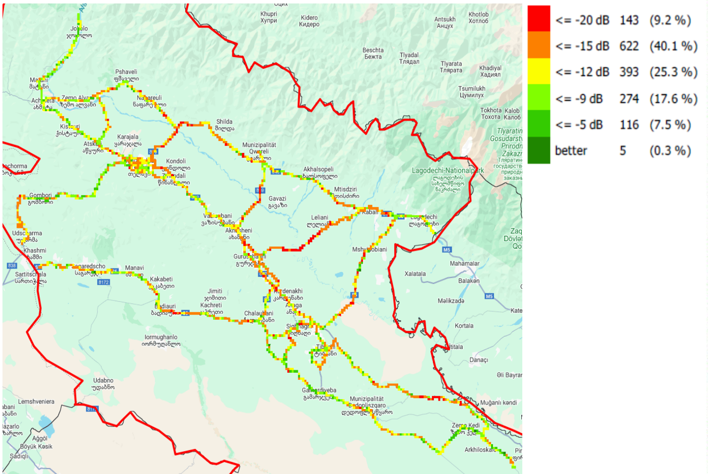
RSRQ, მაგთიკომი
