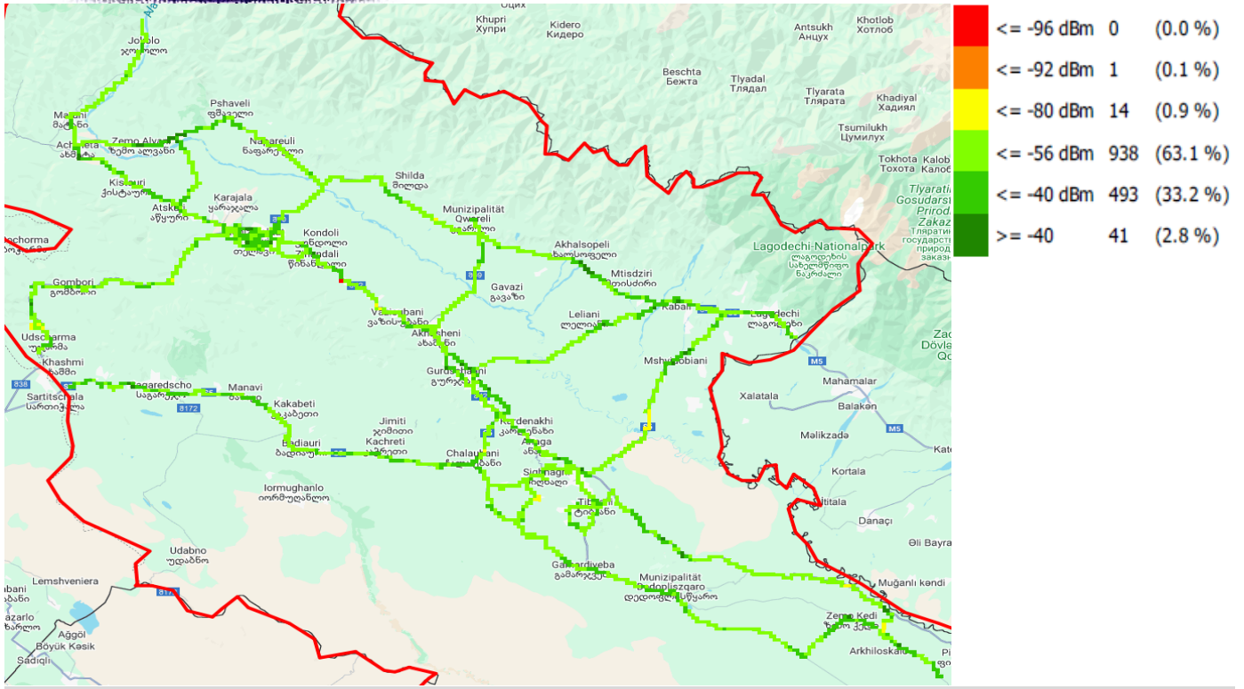
RX_LEV, სილენტი
