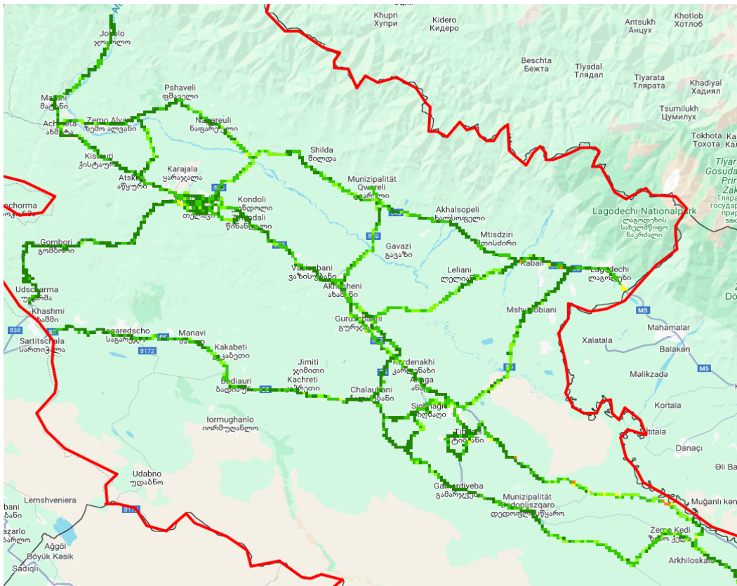
Ec/Io, სილენეტი
