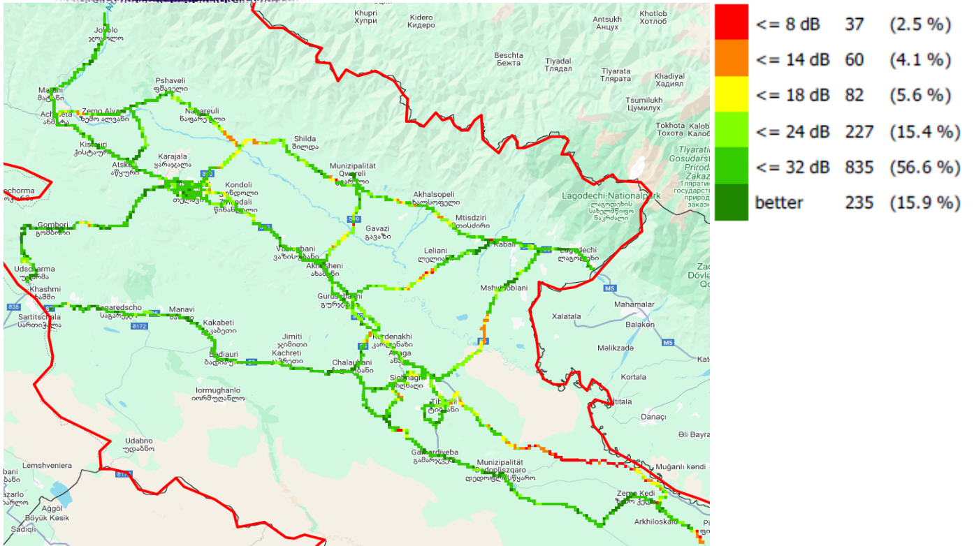
C/I, მგეტიკომი
