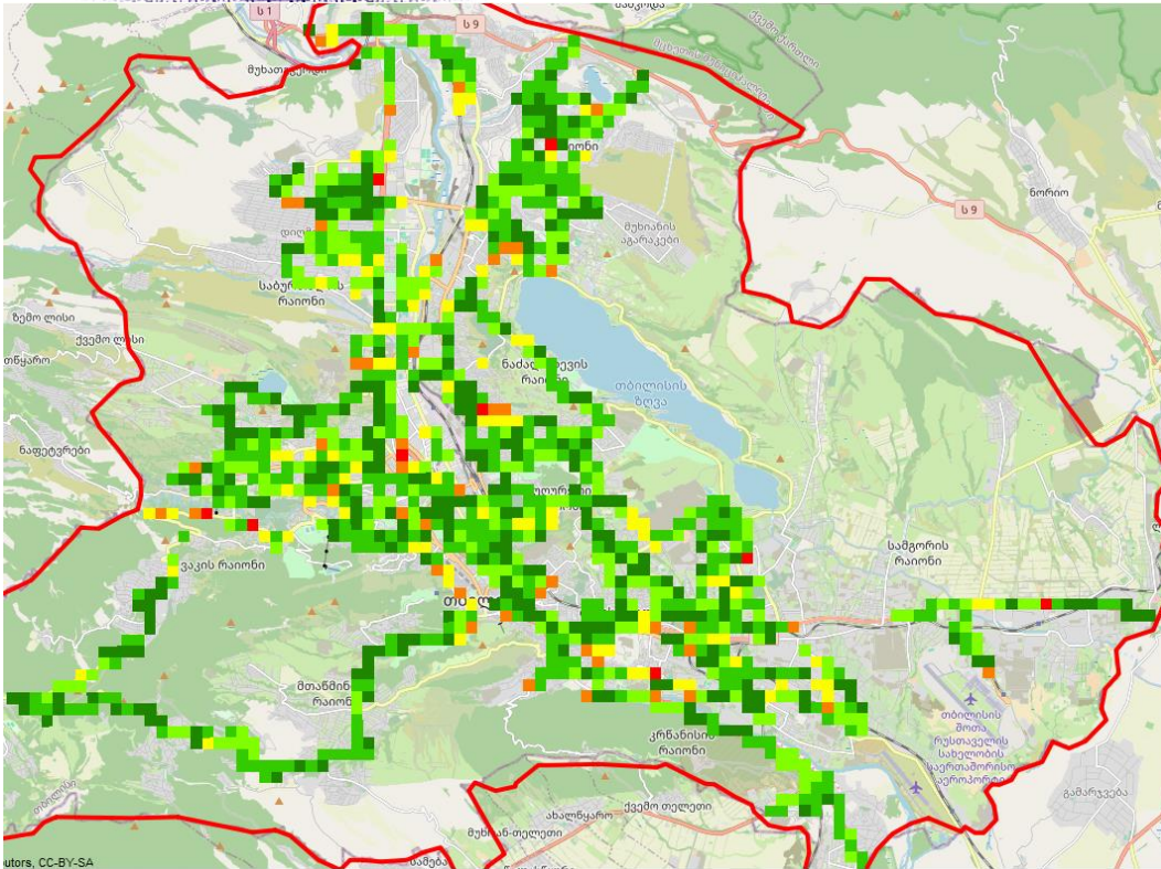
Ec/Io, მაგთიკომი
