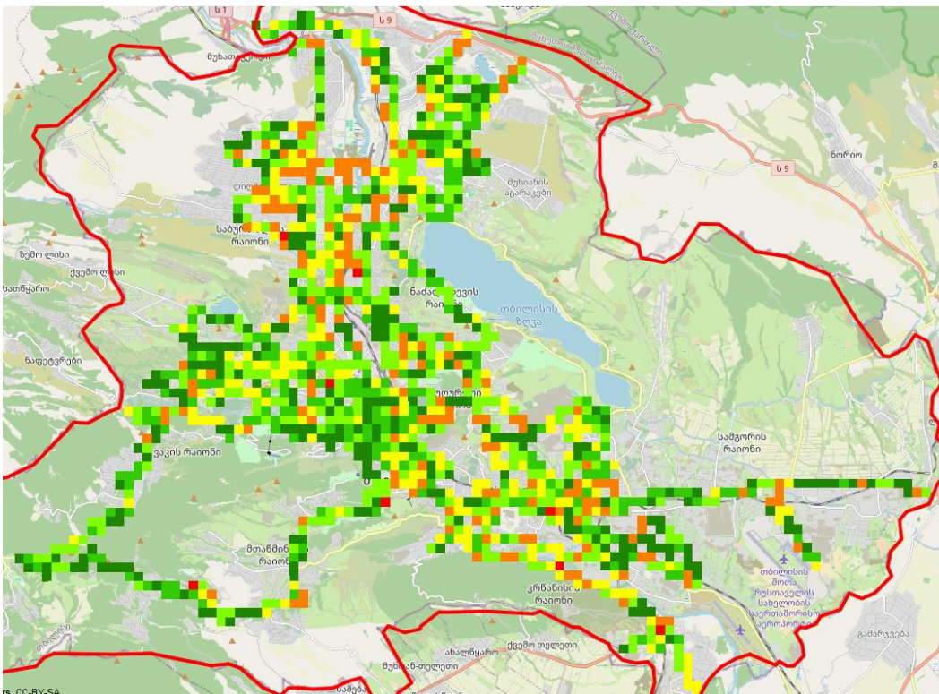
SINR, სილქნეტი
