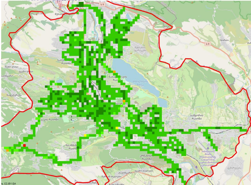
RSRP, სელფი
