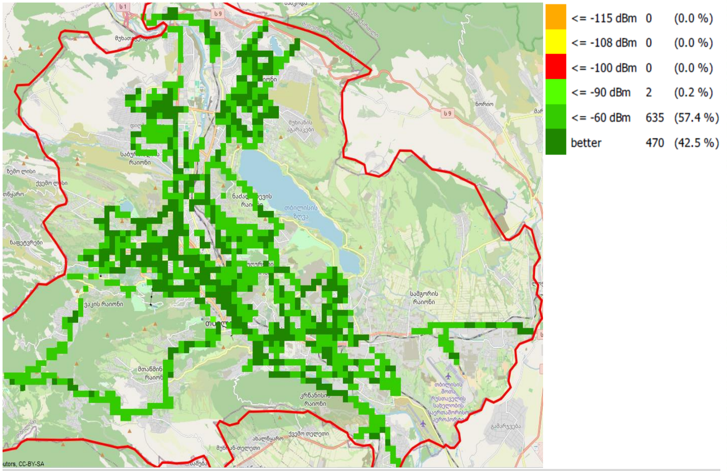
RSCP, მაგთიკომი
