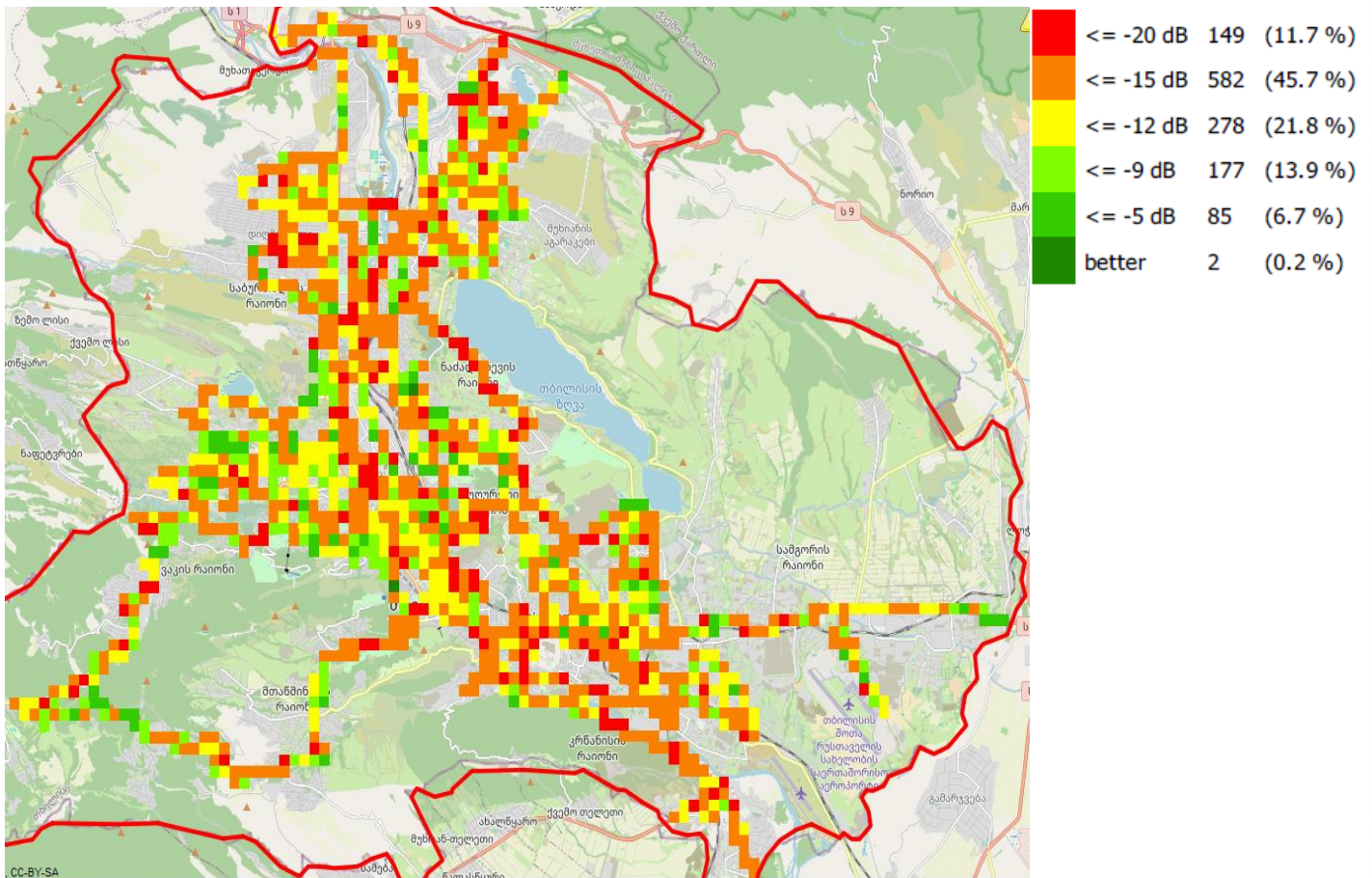
RSRQ, მაგთიკომი
