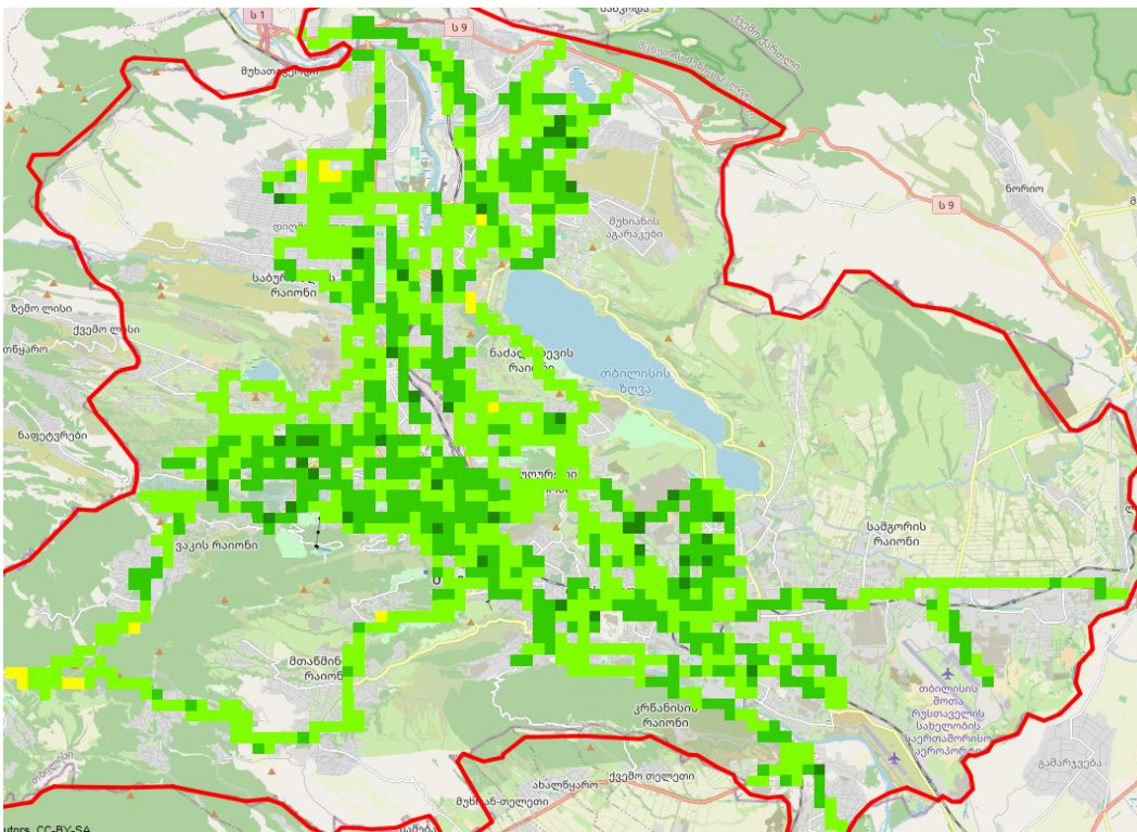
RX_LEV, სელგი
