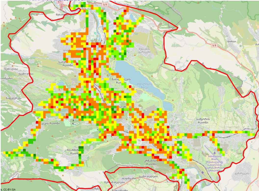
RSRQ, სილქნეტი
