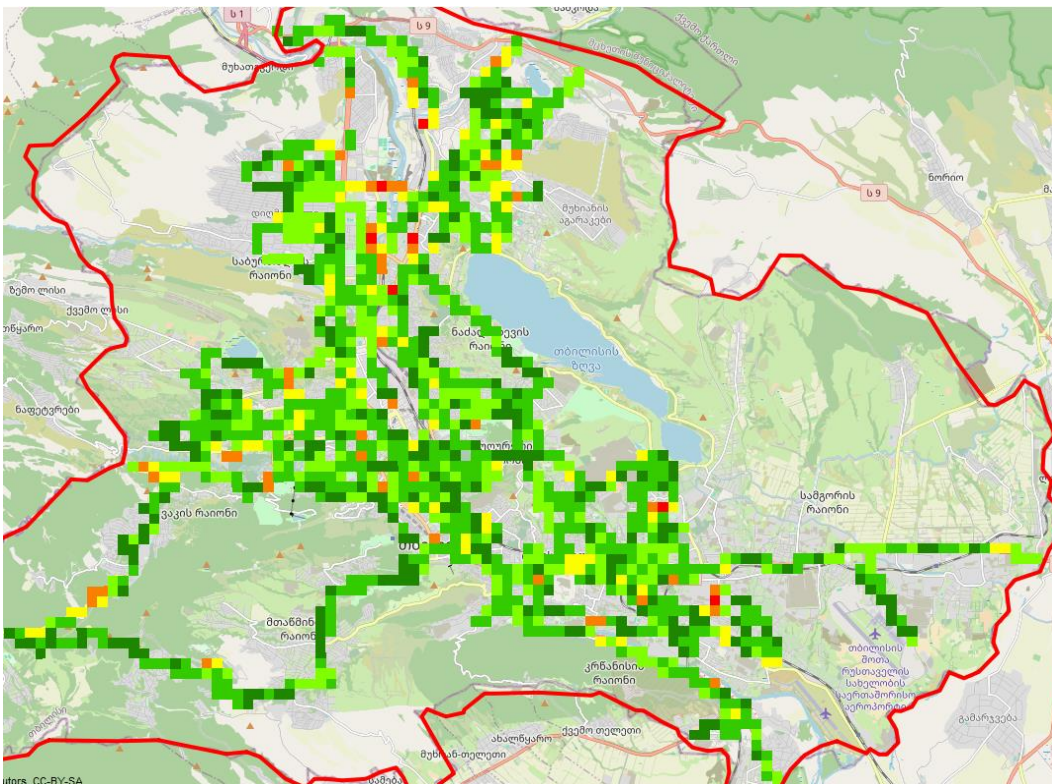
Ec/Io, სილქნეტი
