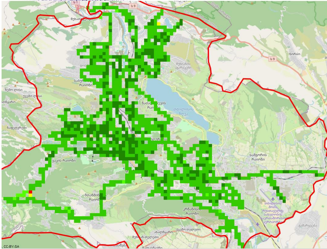
RSRP, მაგთიკომი
