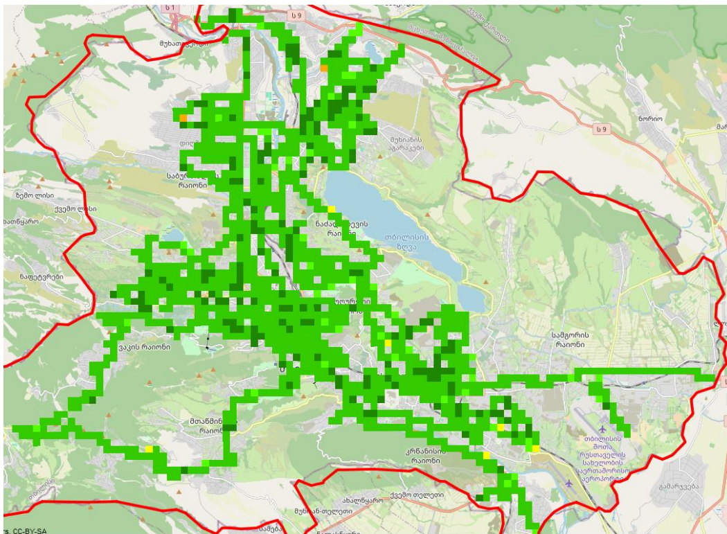
RSRP, სილქნეტი
