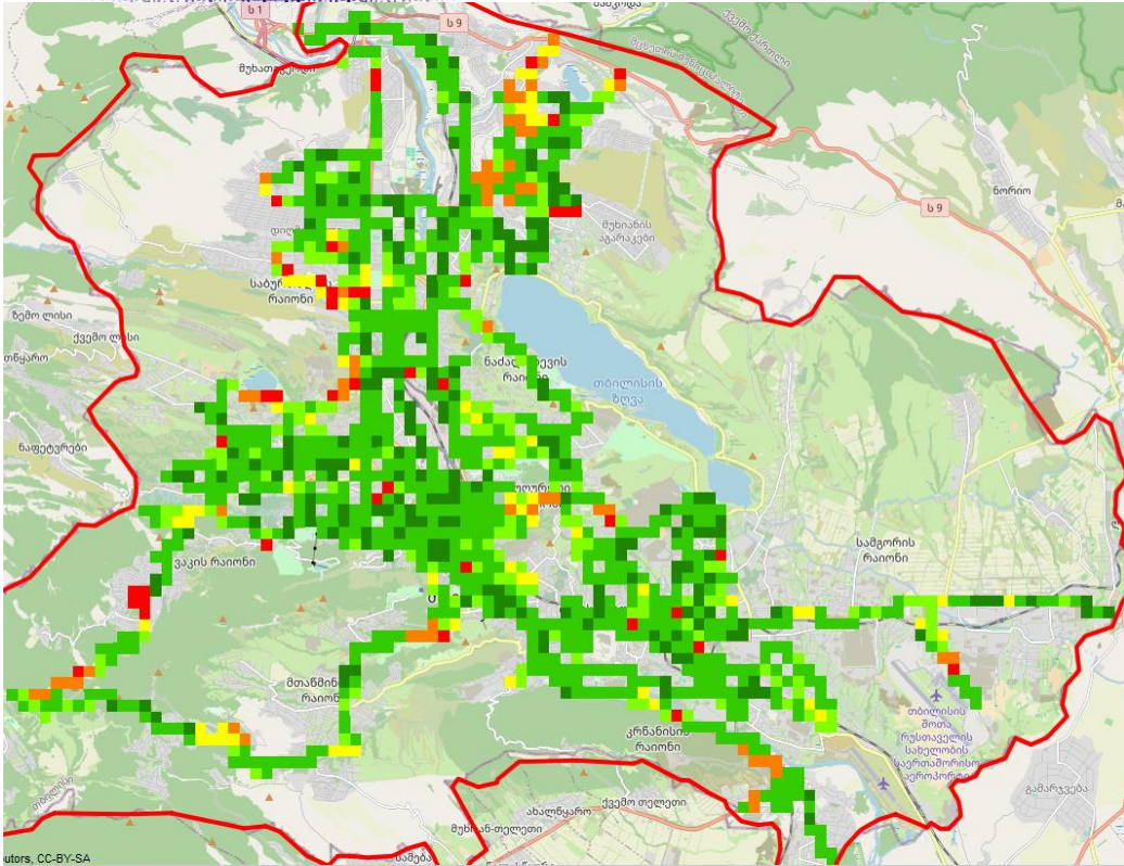
C/I, მაგთიკომი
