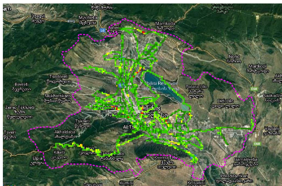
RSCP, მაგთიკომი
