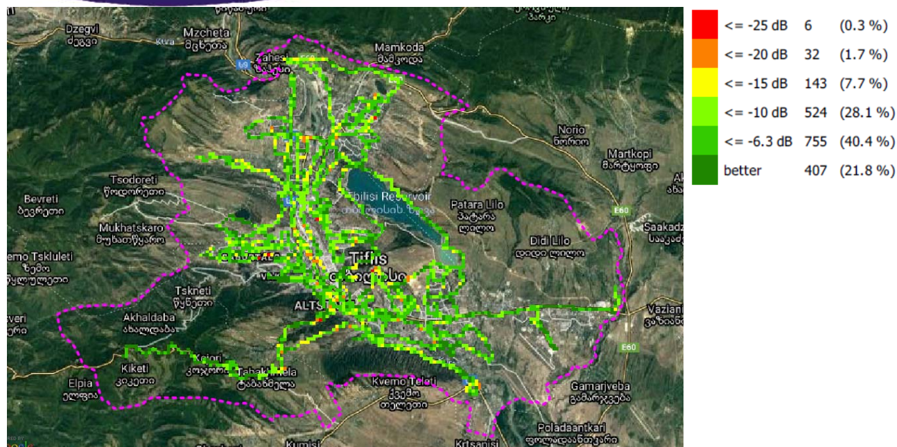
Ec/Io, სილქნეტი
