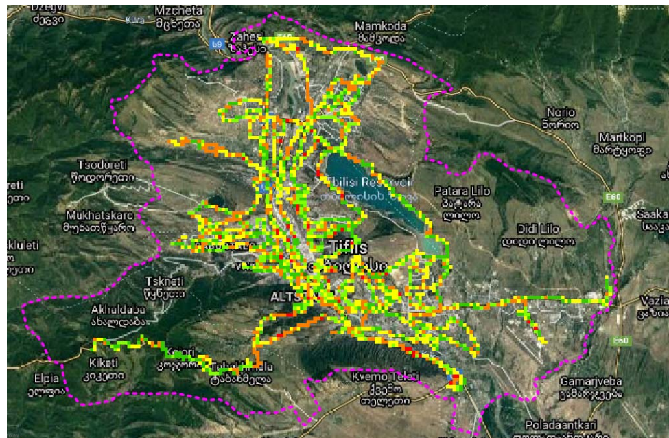
RSRQ, სილქნეტი
