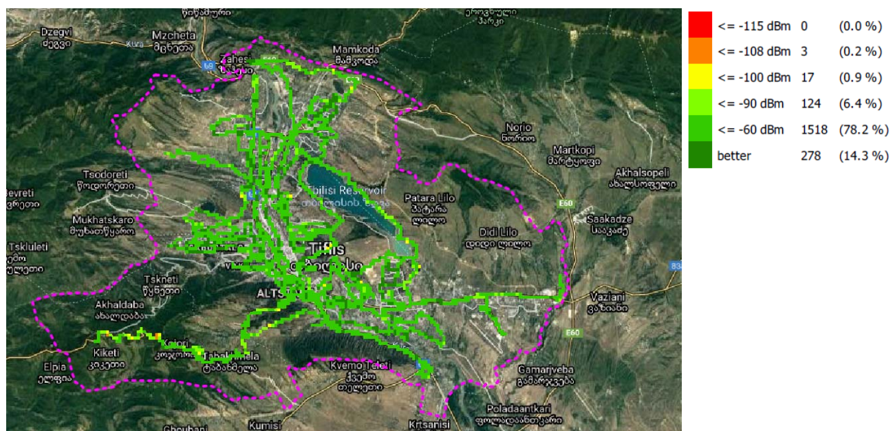
RSRP, ვიონ საქართველო
