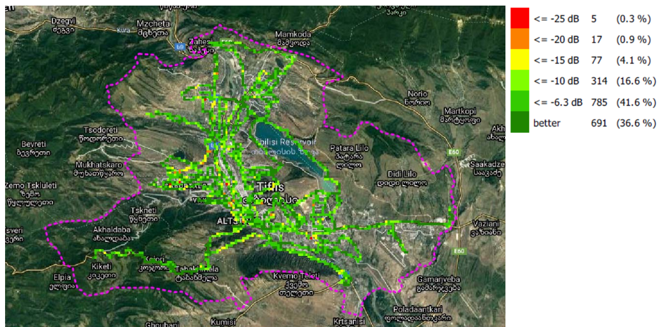
Ec/Io, ვიონი საქართველო
