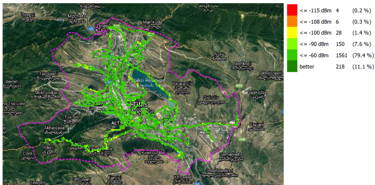
RSRP, სილქნეტი
