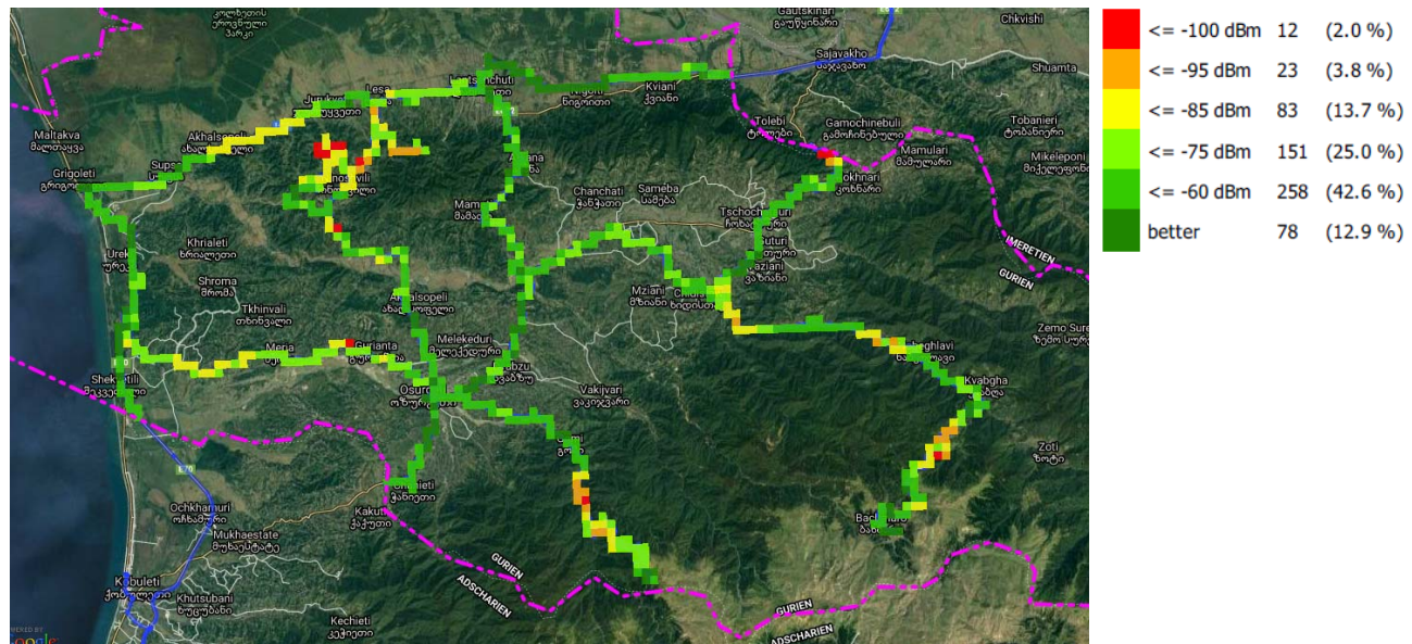
RSCP, მაგთიკომი
