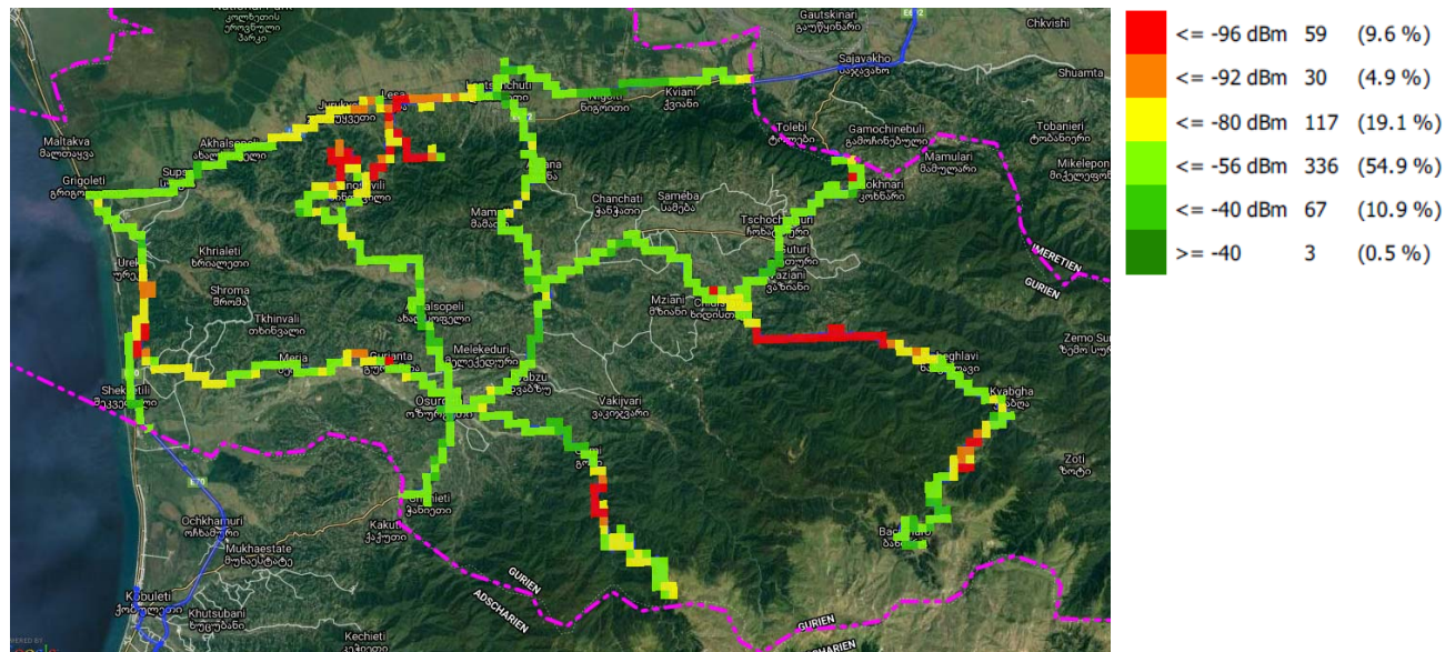
RX_LEV, ვიონი საქართველო
