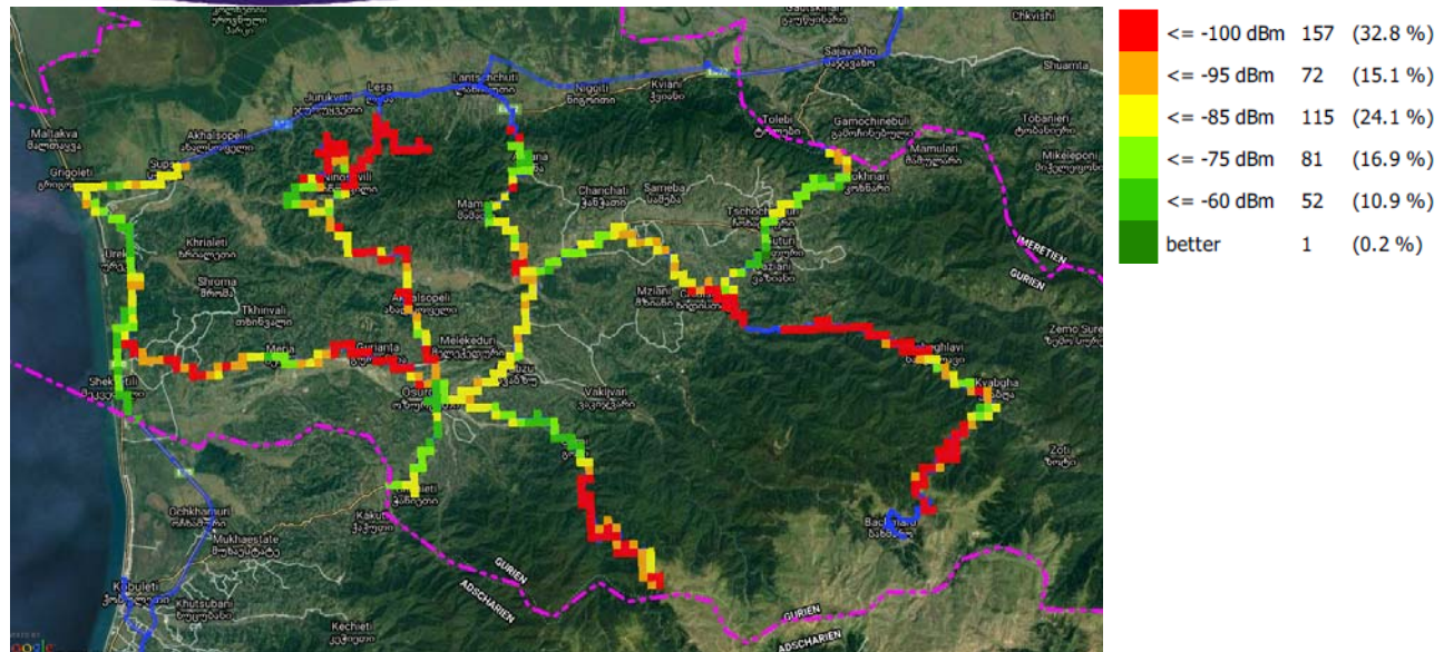
RSCP, ვიონი საქართველო
