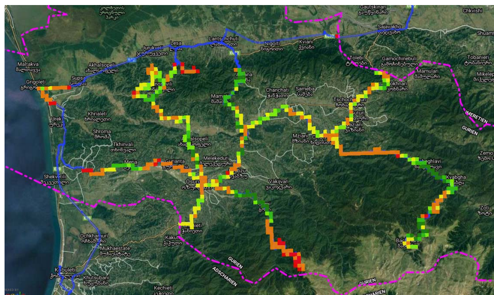
SINR, ვიონი საქართველო
