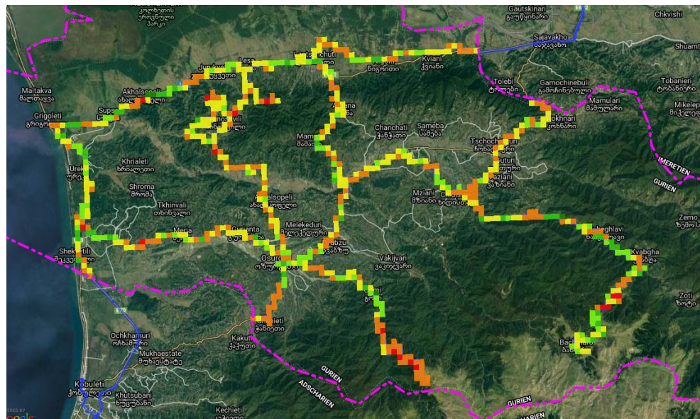
RSRQ, სილენეტი
