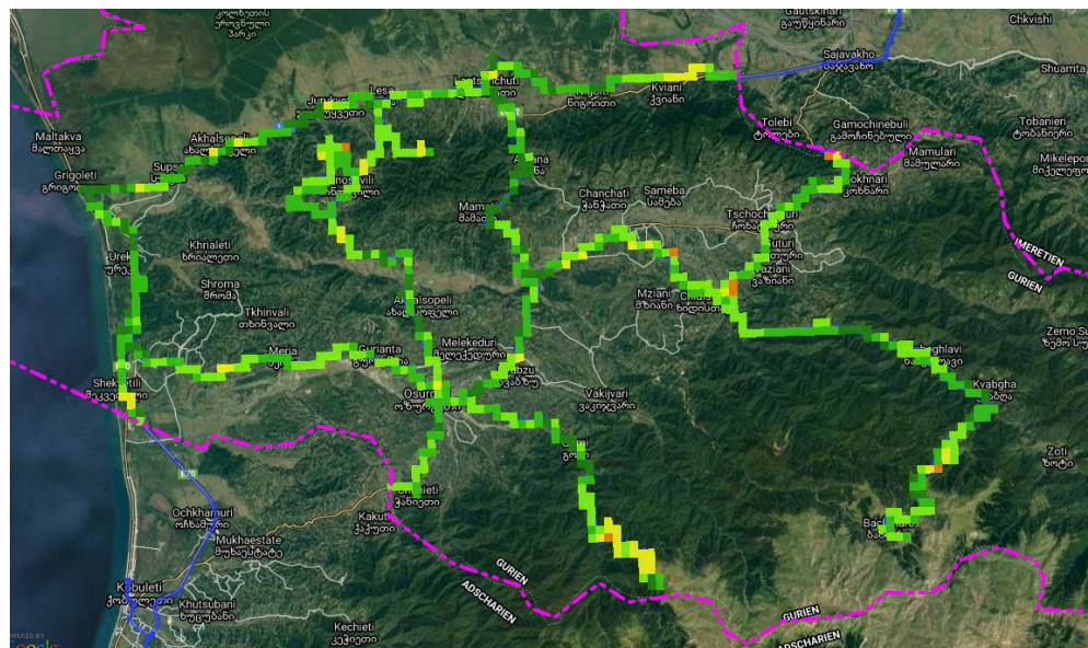
Ec/Io, მაგთიკომი
