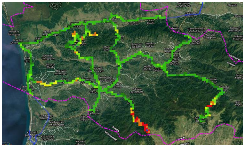
C/I, სილქნეტი
