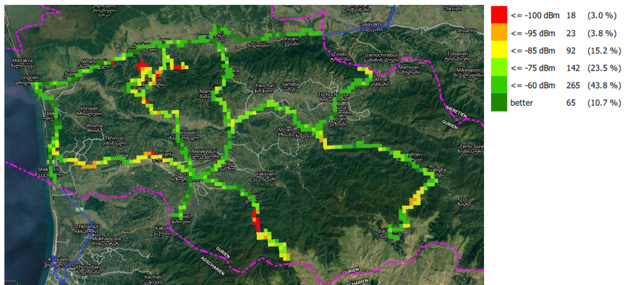
RSCP, სილქნეტი
