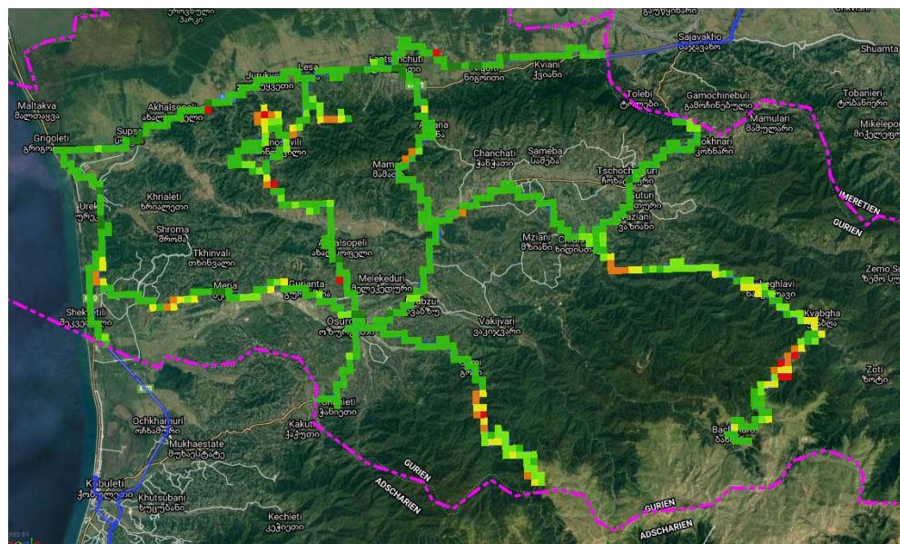
RSRP, სილქნეტი
