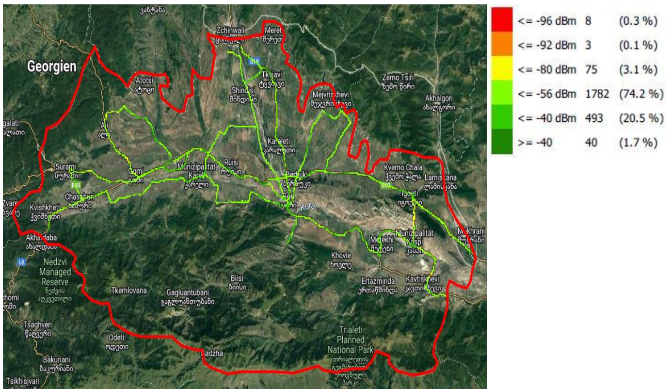
RX_LEV, ვიონი საქართველო
