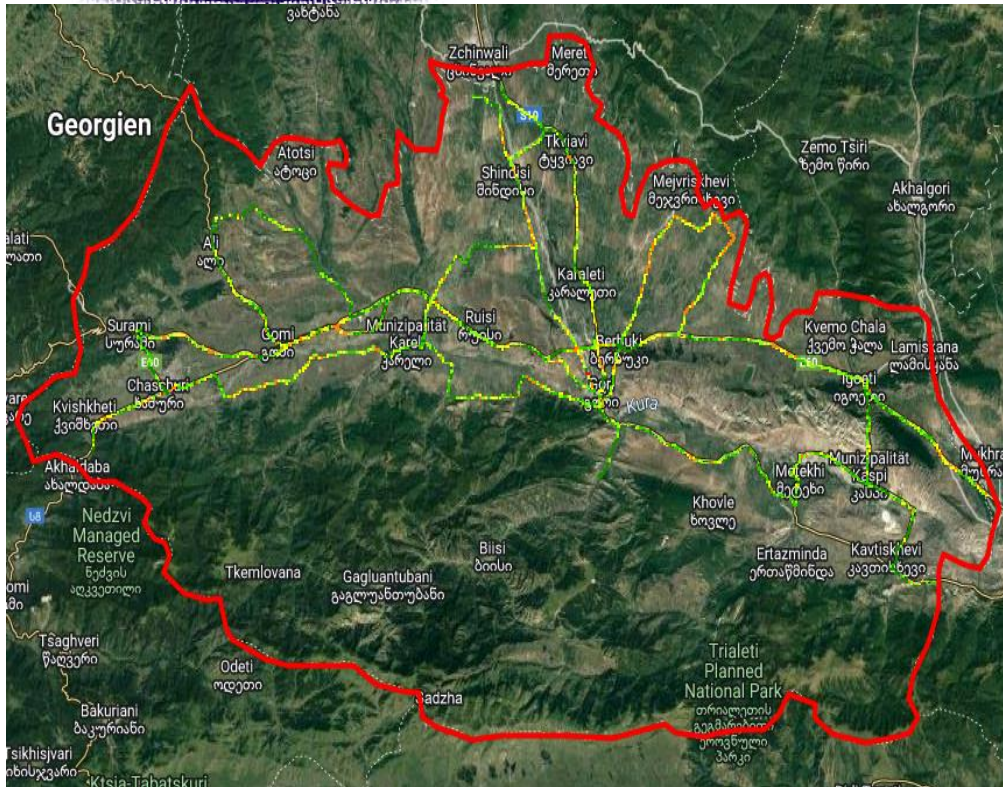
SINR, სილქნეტი
