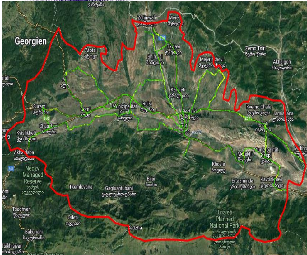
RSCP, სილქნეტი
