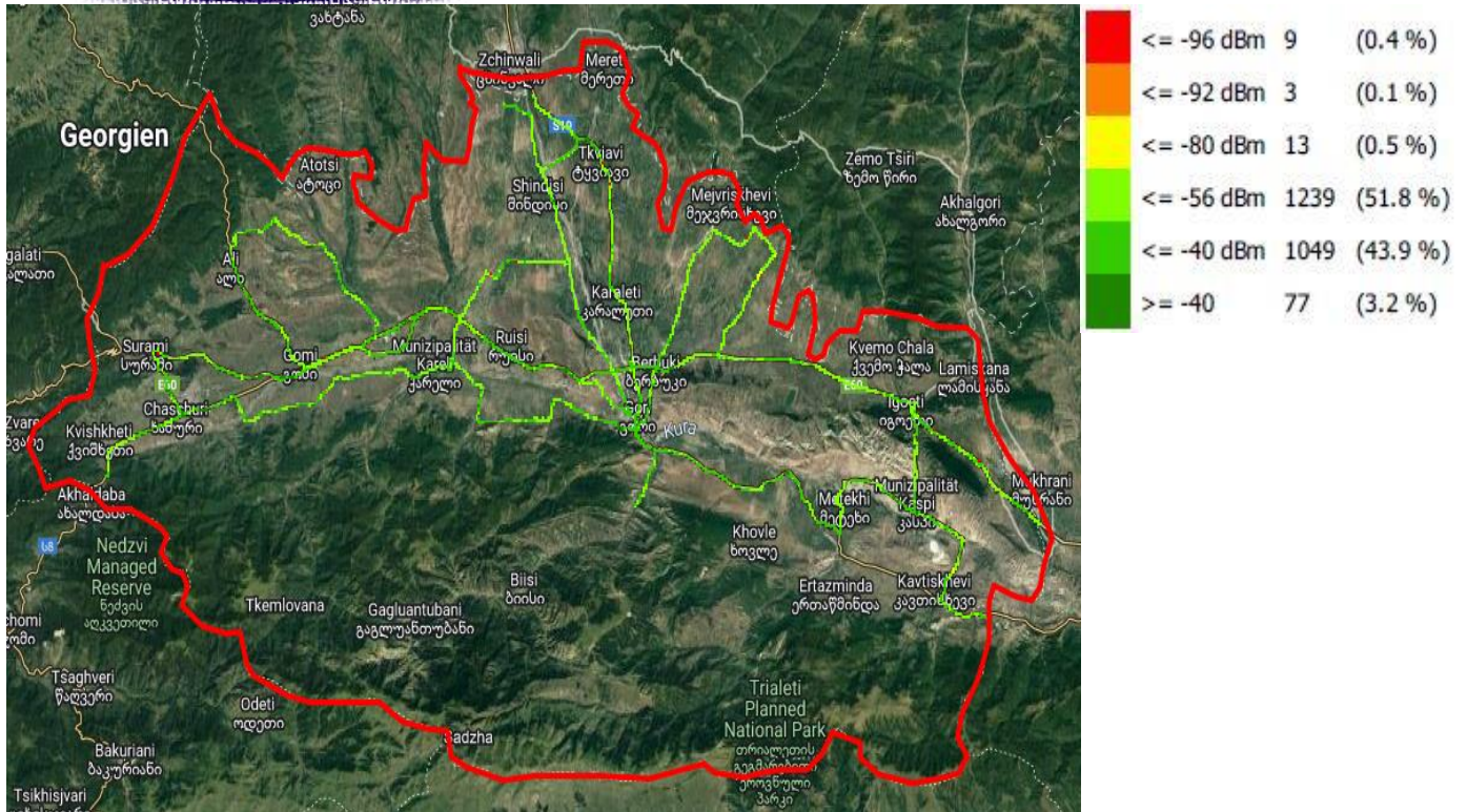
RX_LEV, სილქნეტი
