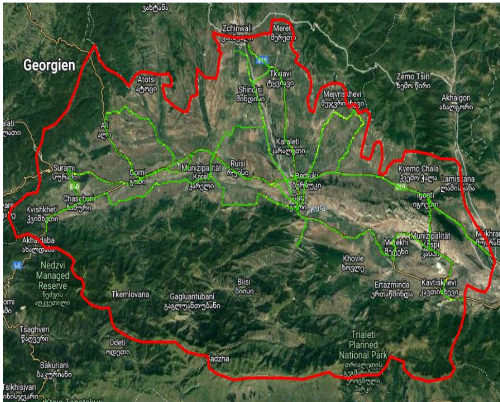
RSRP, სილქნეტი
