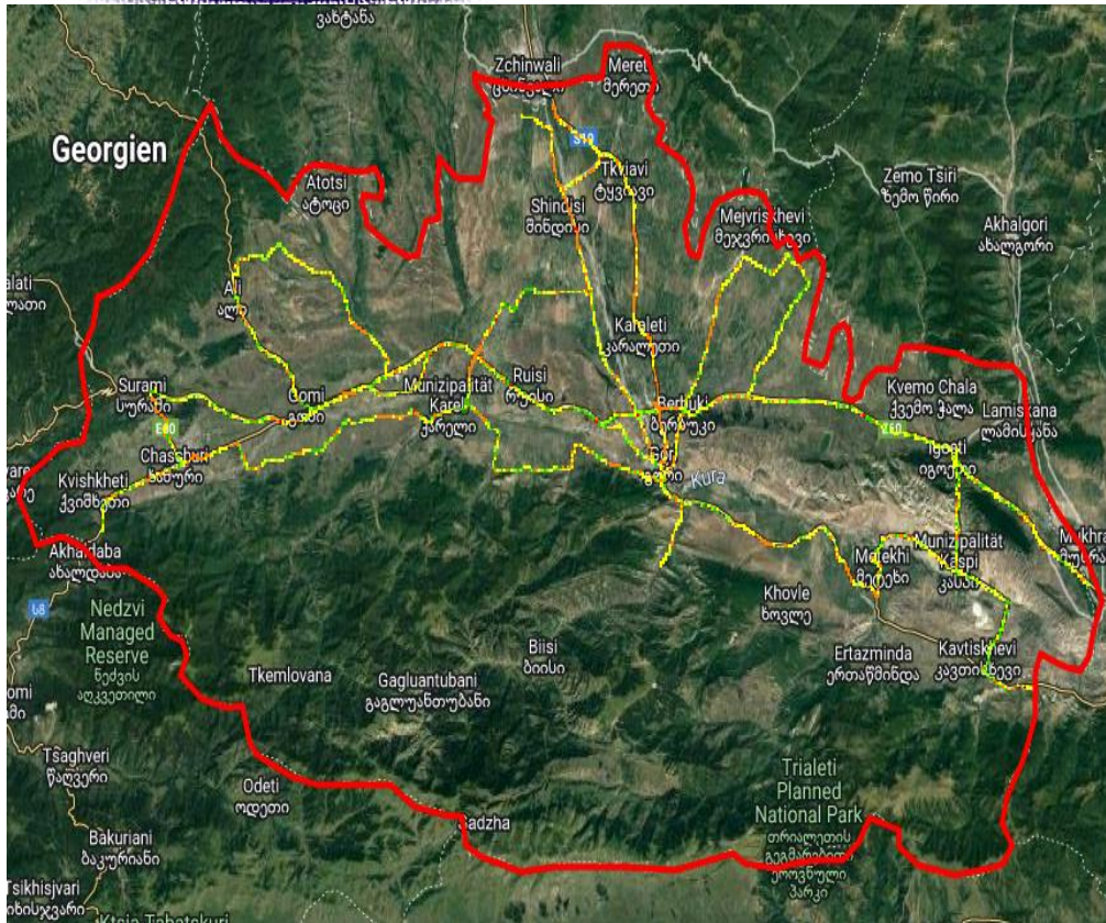
RSRQ, მაგთიკომი
