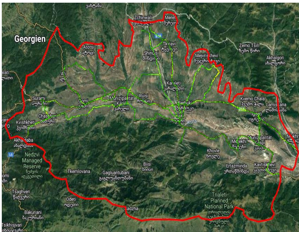
Ec/Io, მაგნიტუდა
