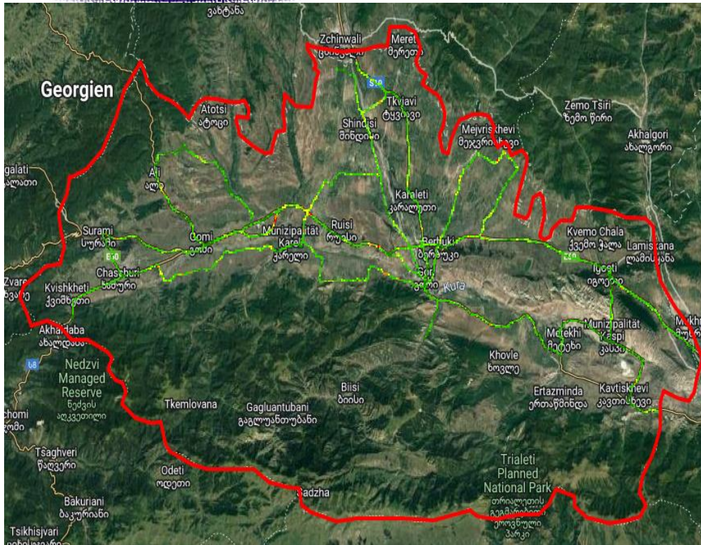
C/I, მაგთიკომი
