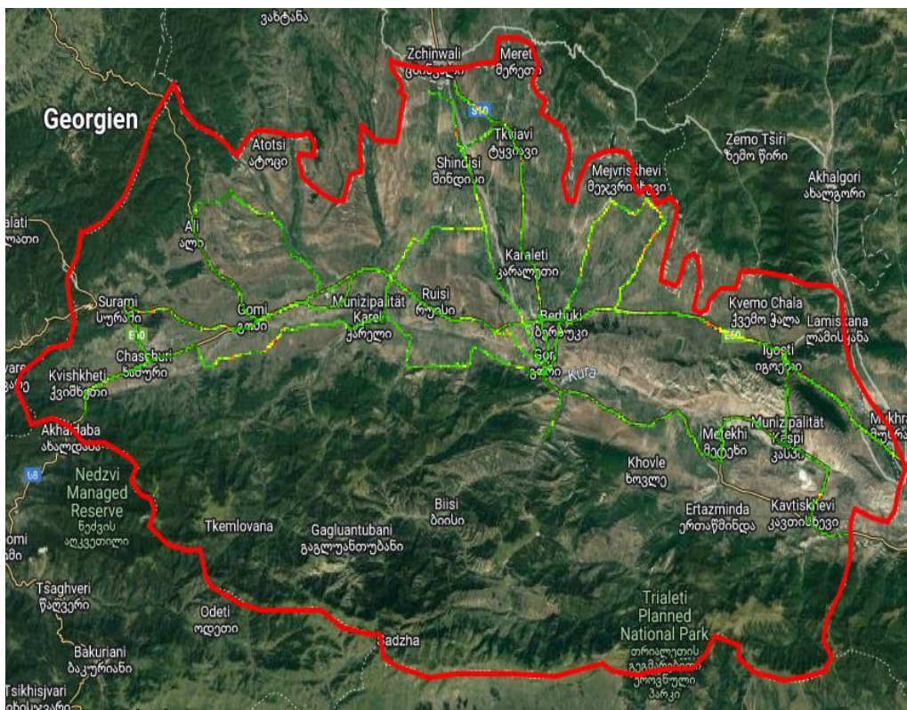
C/I, სილქნეტი
