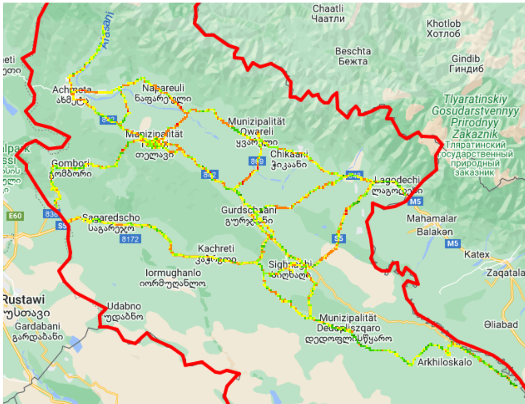
RSRQ, მაგთიკომი
