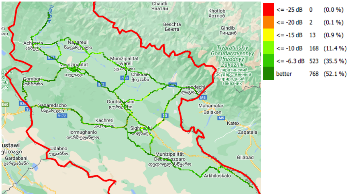
EC/Io, სილქნეტი
