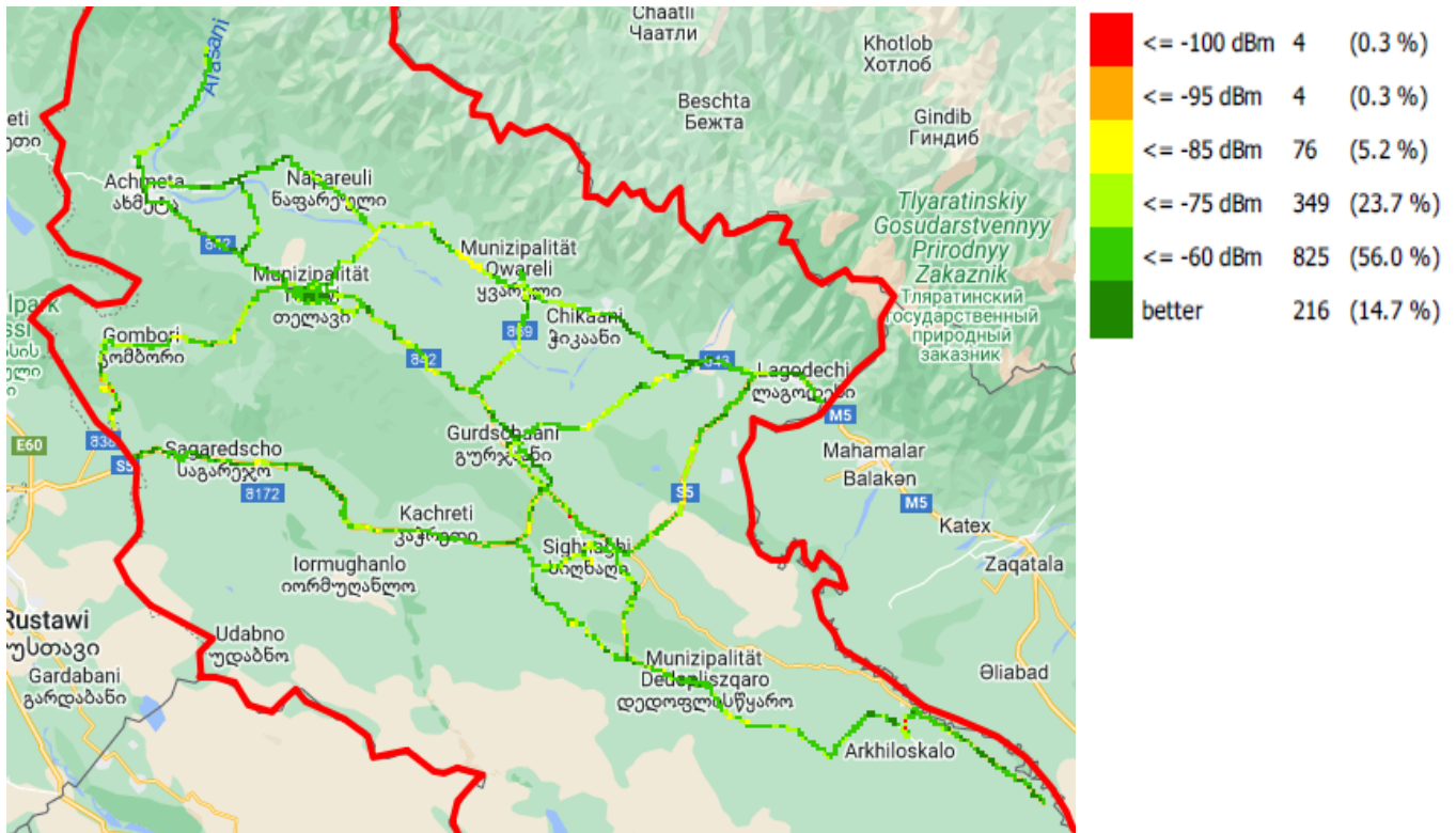
RSCP, სილქნეტი
