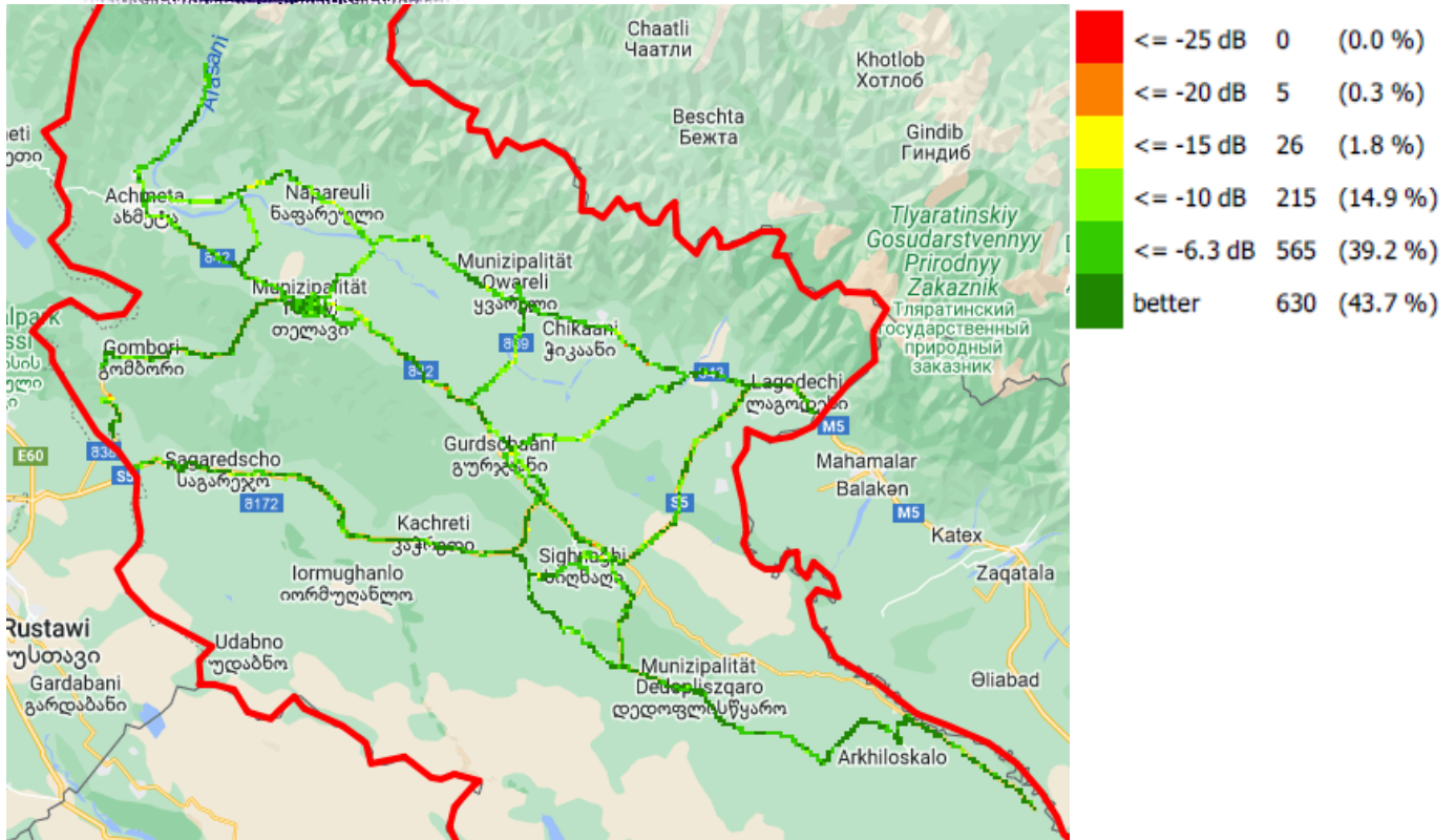
EC/Io, მათეკომი
