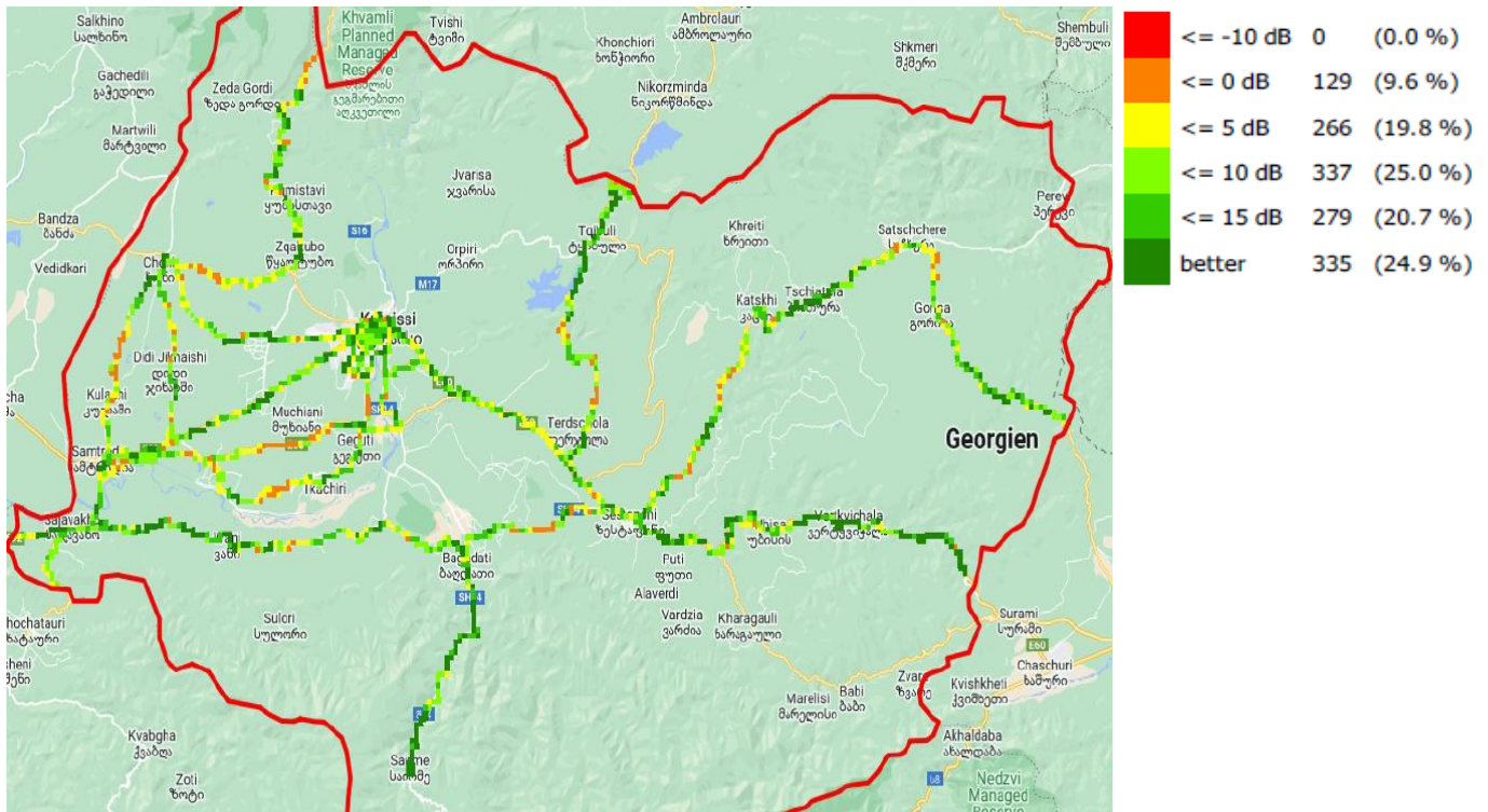
SINR, სილქნეტი
