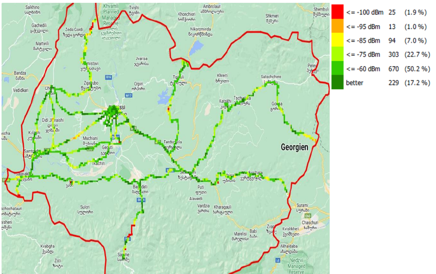
RSCP, მაგთიკომი
