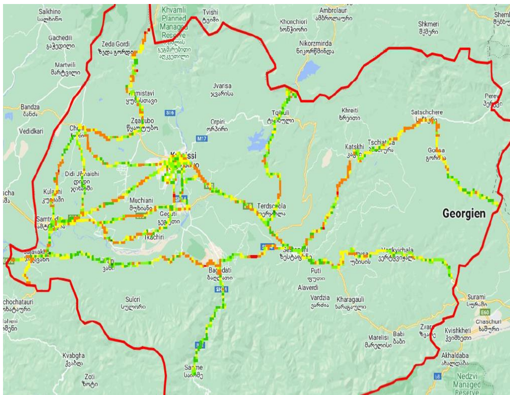
RSRQ, სილქნეტი
