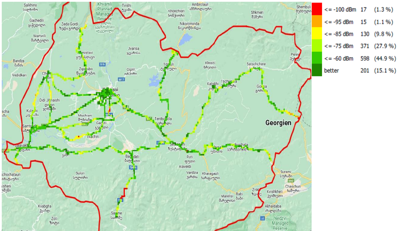
RSCP, სილქნეტი
