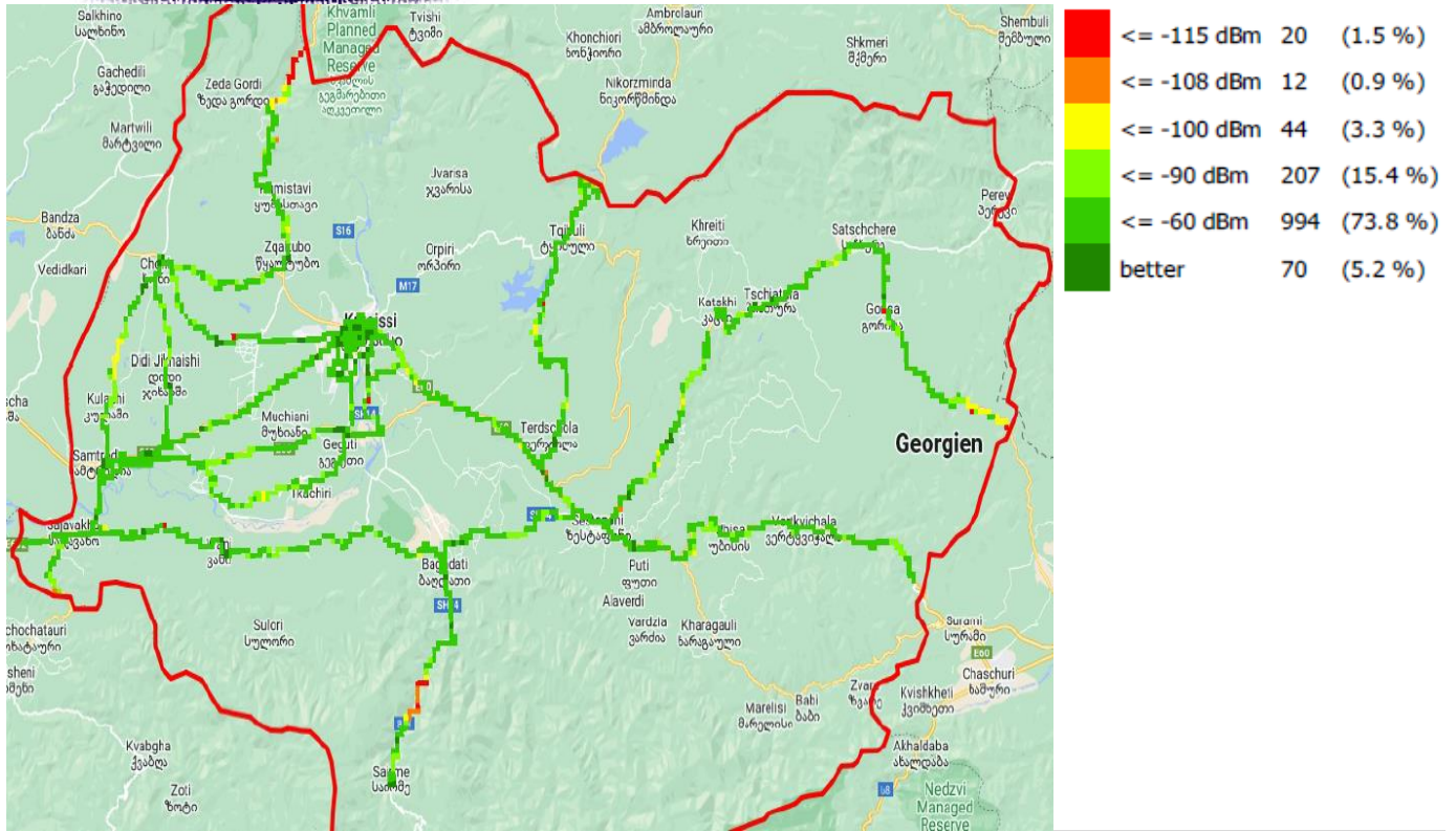
RSRP, სოლქნეტი
