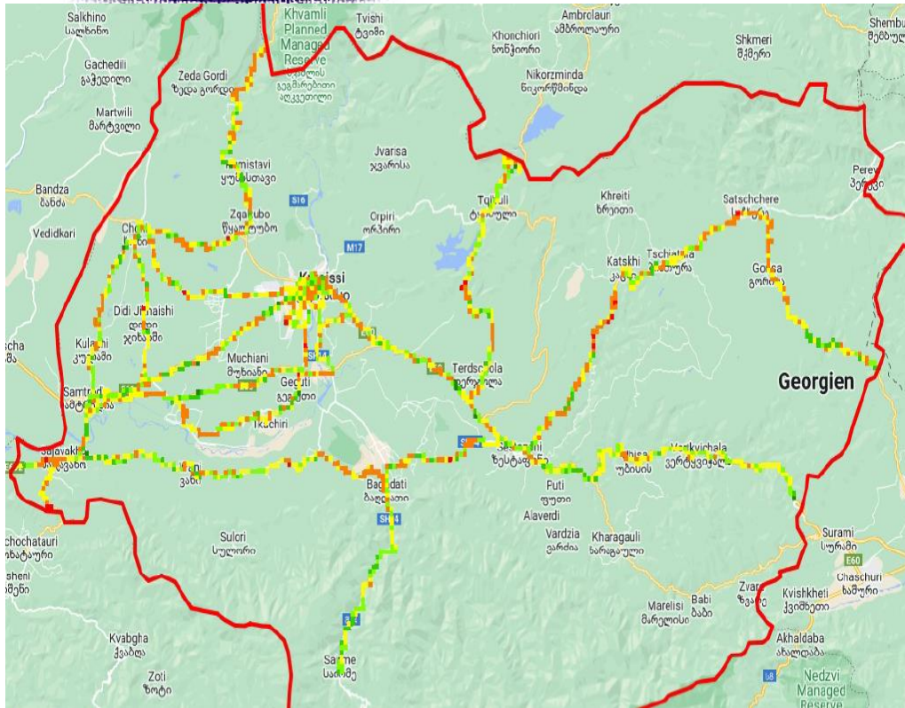
RSRQ, მაგთიკომი
