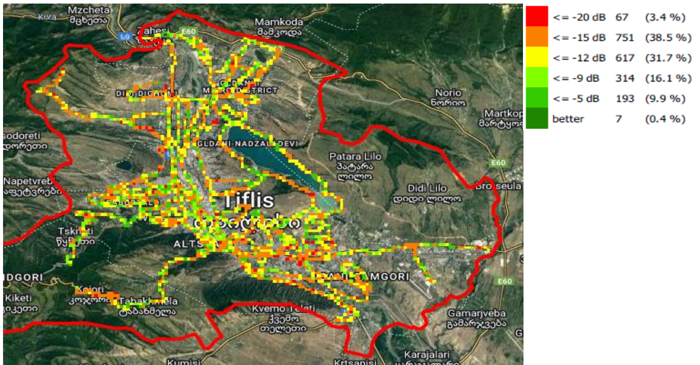
RSRQ ვიონი საქართველო
