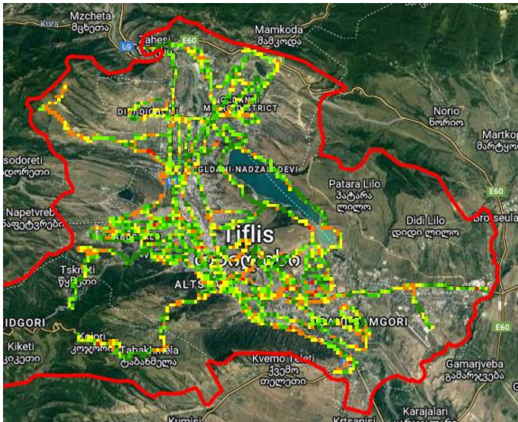
SINR, ვიონი საქართველო
